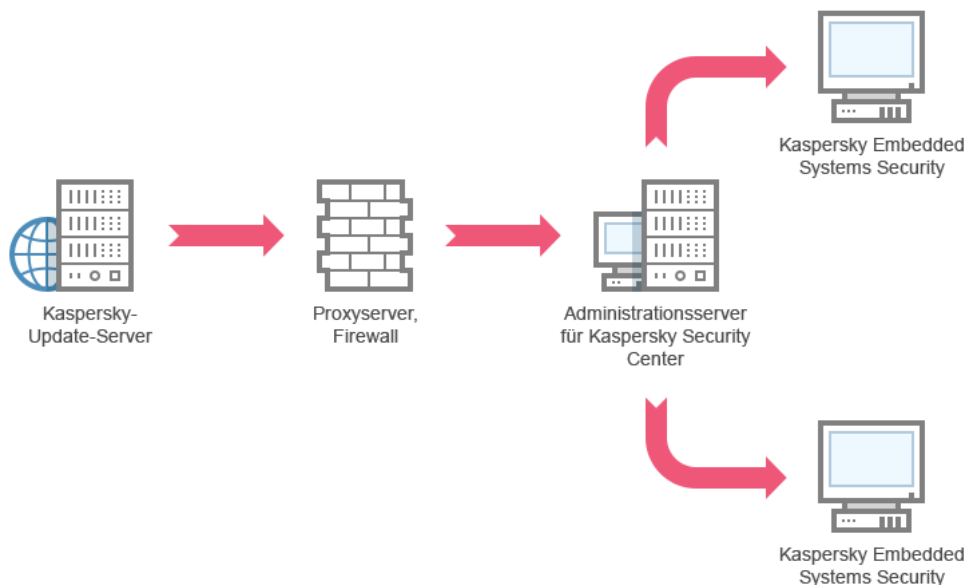
Abbildung 3: Aktualisieren von Datenbanken und Modulen über einen Kaspersky Security Center-Administrationsserver
