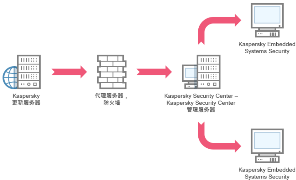
方案 3: 通过 Kaspersky Security Center 管理服务器更新数据库和模块
