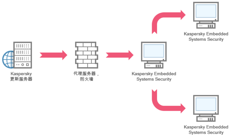
方案 2: 通过一个受保护设备更新数据库和模块
