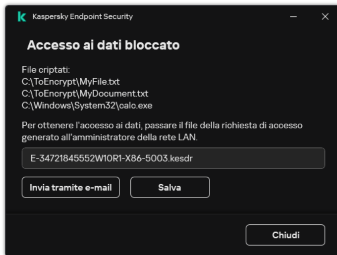
Richiesta di accesso ai dati criptati
