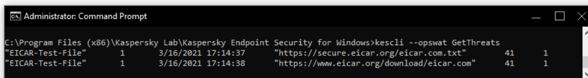
Gestione dell'applicazione dalla riga di comando
