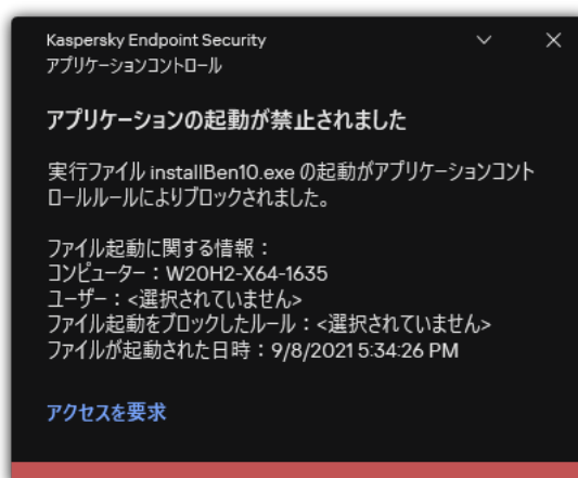
実行防止の通知
