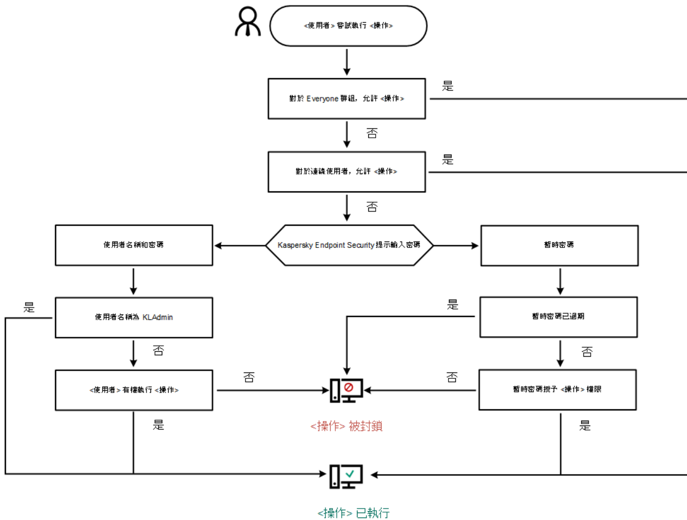
密碼防護操作演算法
