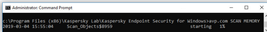
Gestionarea aplicației din linia de comandă
