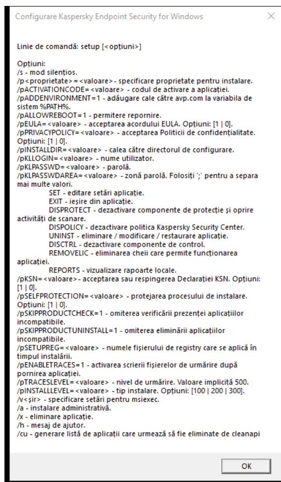
Descrierea opțiunilor comenzii de instalare
