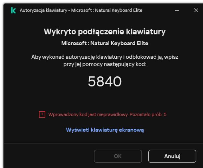
Autoryzacja klawiatury
