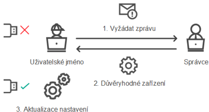
Schéma pro udělení přístupu k zařízení v režimu online
