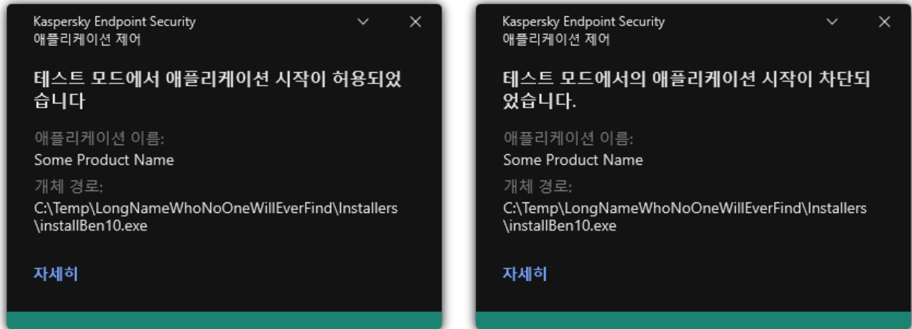
테스트 모드의 애플리케이션 제어 알림
