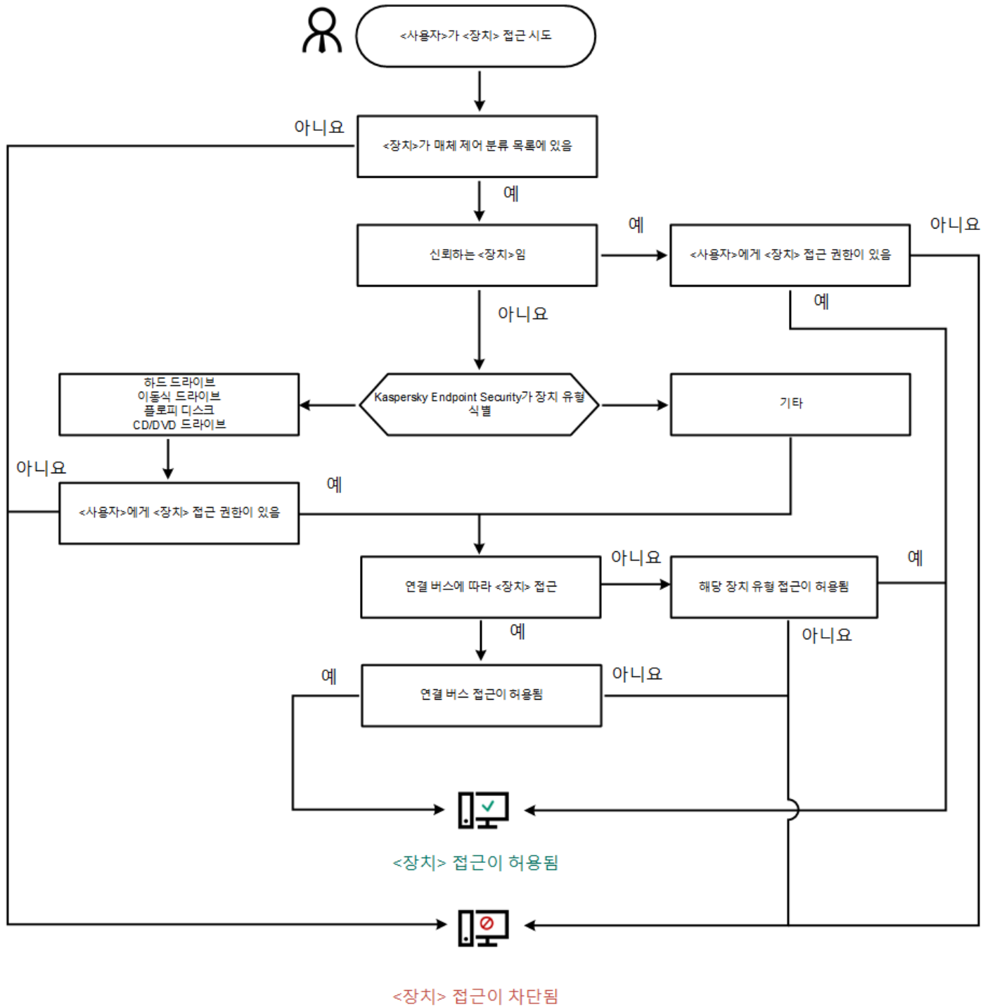
장치 제어 동작 알고리즘
