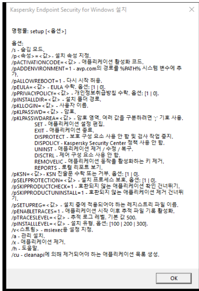
설치 명령 옵션 설명
