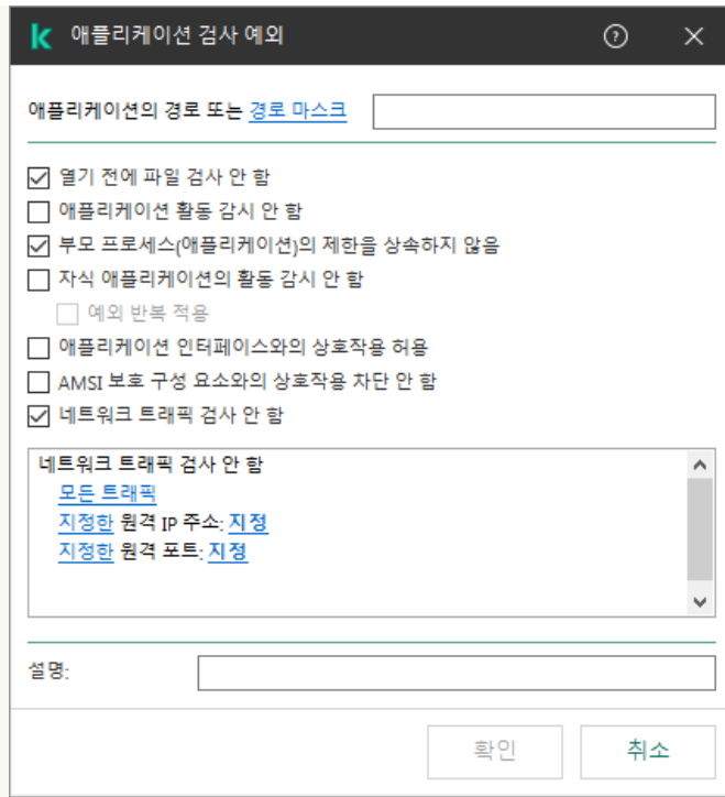
신뢰하는 애플리케이션 설정
