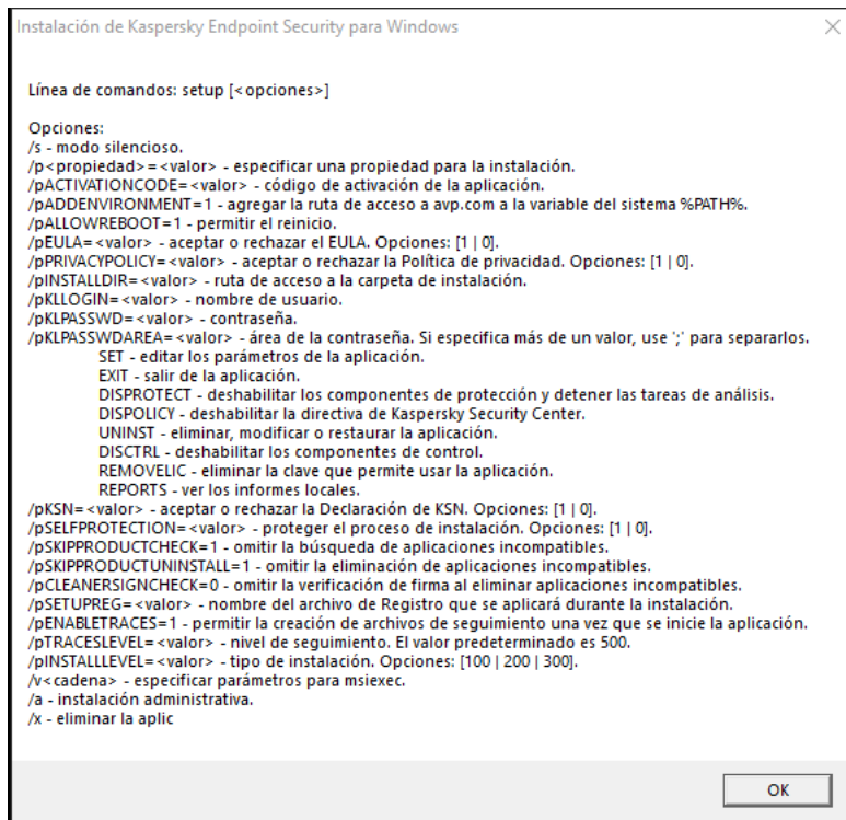
Descripción de las opciones del comando de instalación
