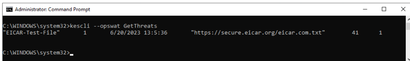
Administración de la aplicación desde la línea de comandos
