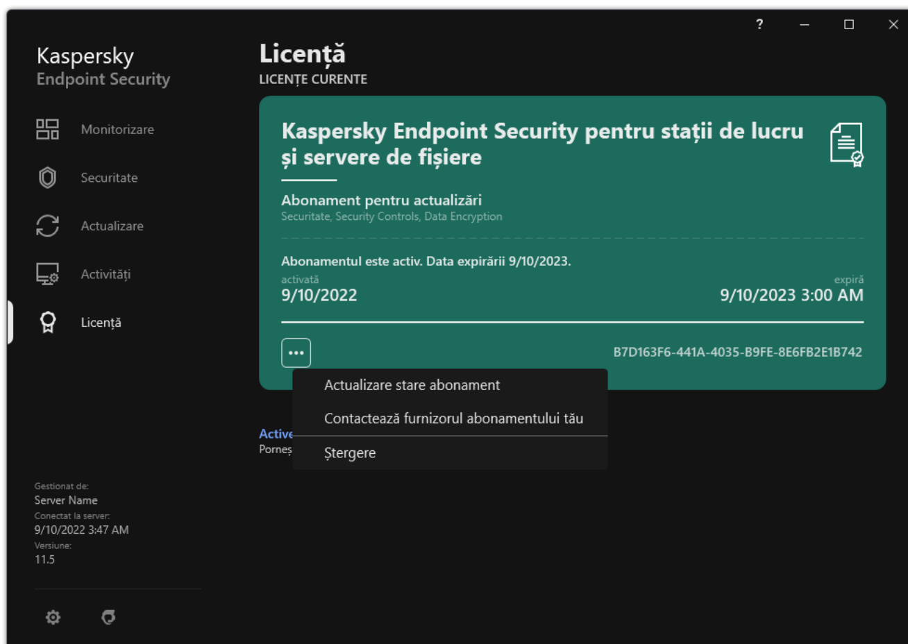
Reînnoirea abonamentului
