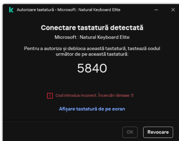
Autorizare tastatură
