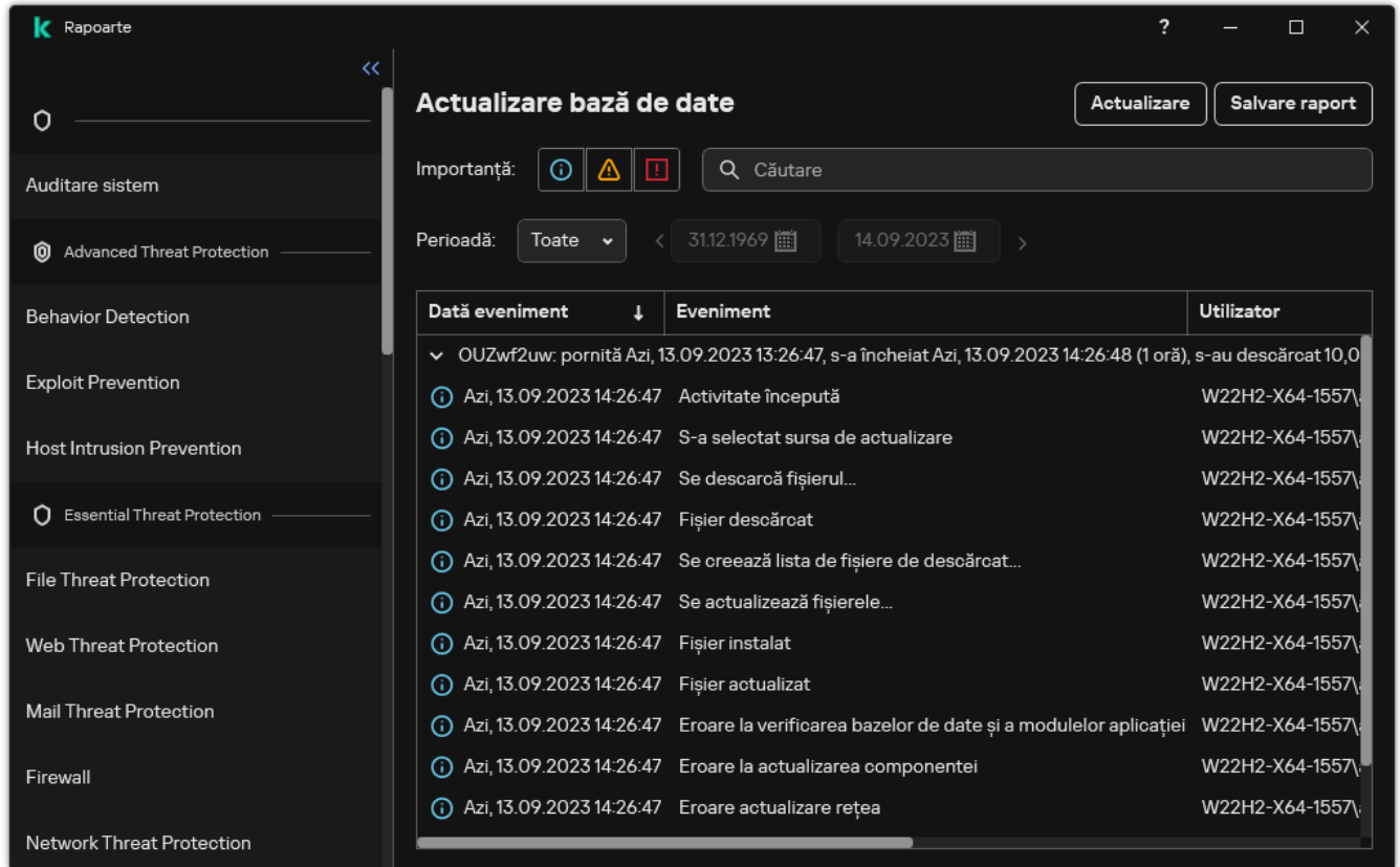
Rapoarte
