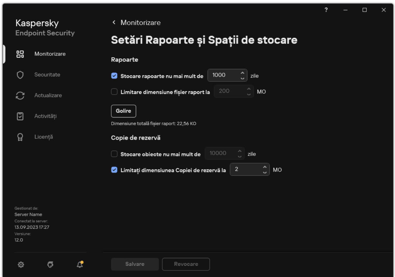
Setări rapoarte
