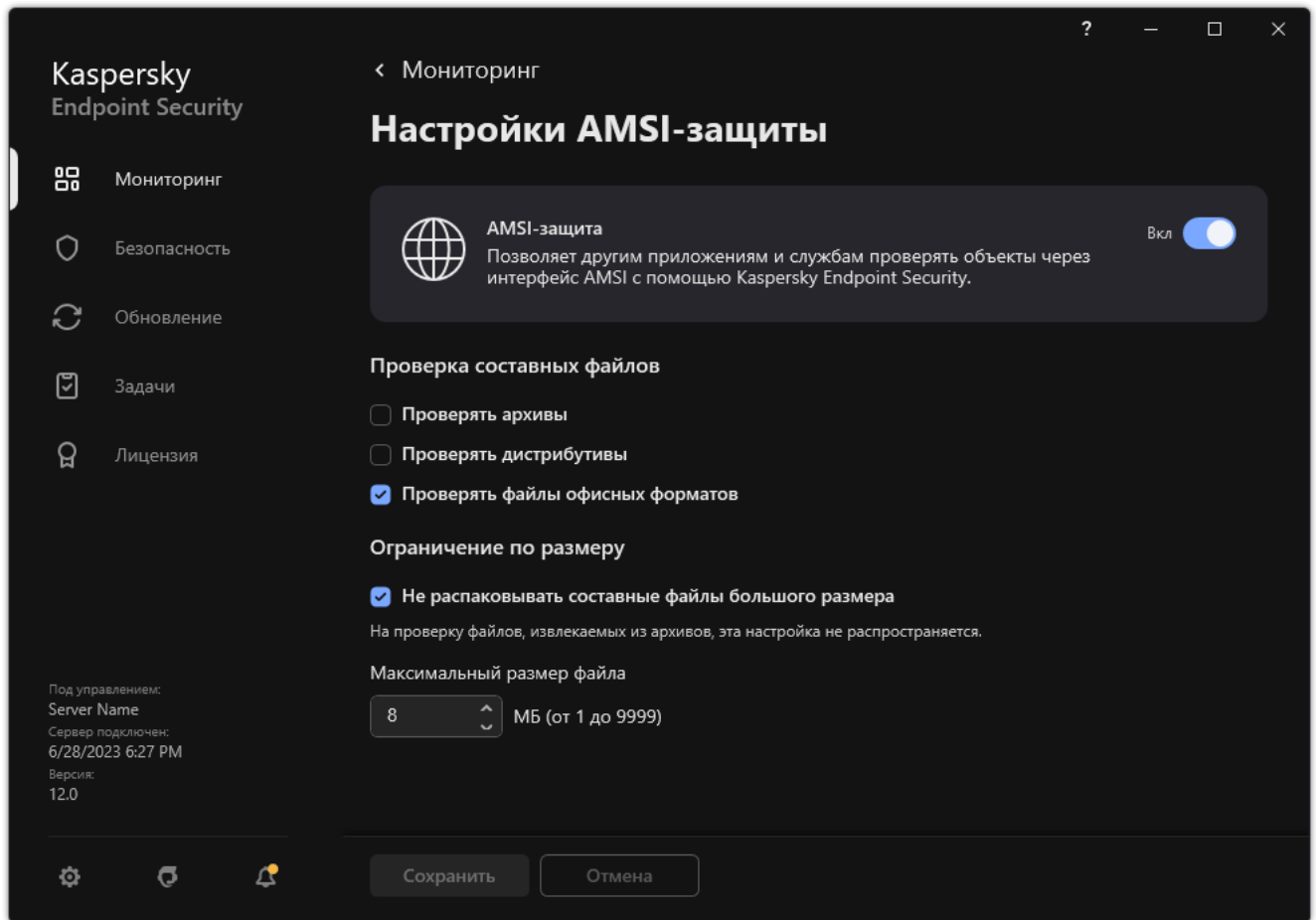
Параметры AMSI-защиты
