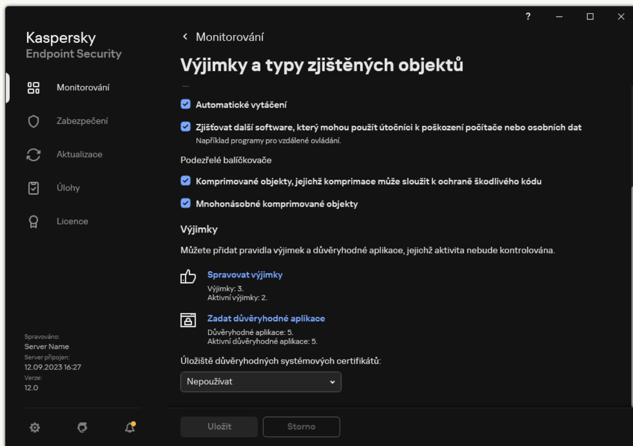
Nastavení výjimek
