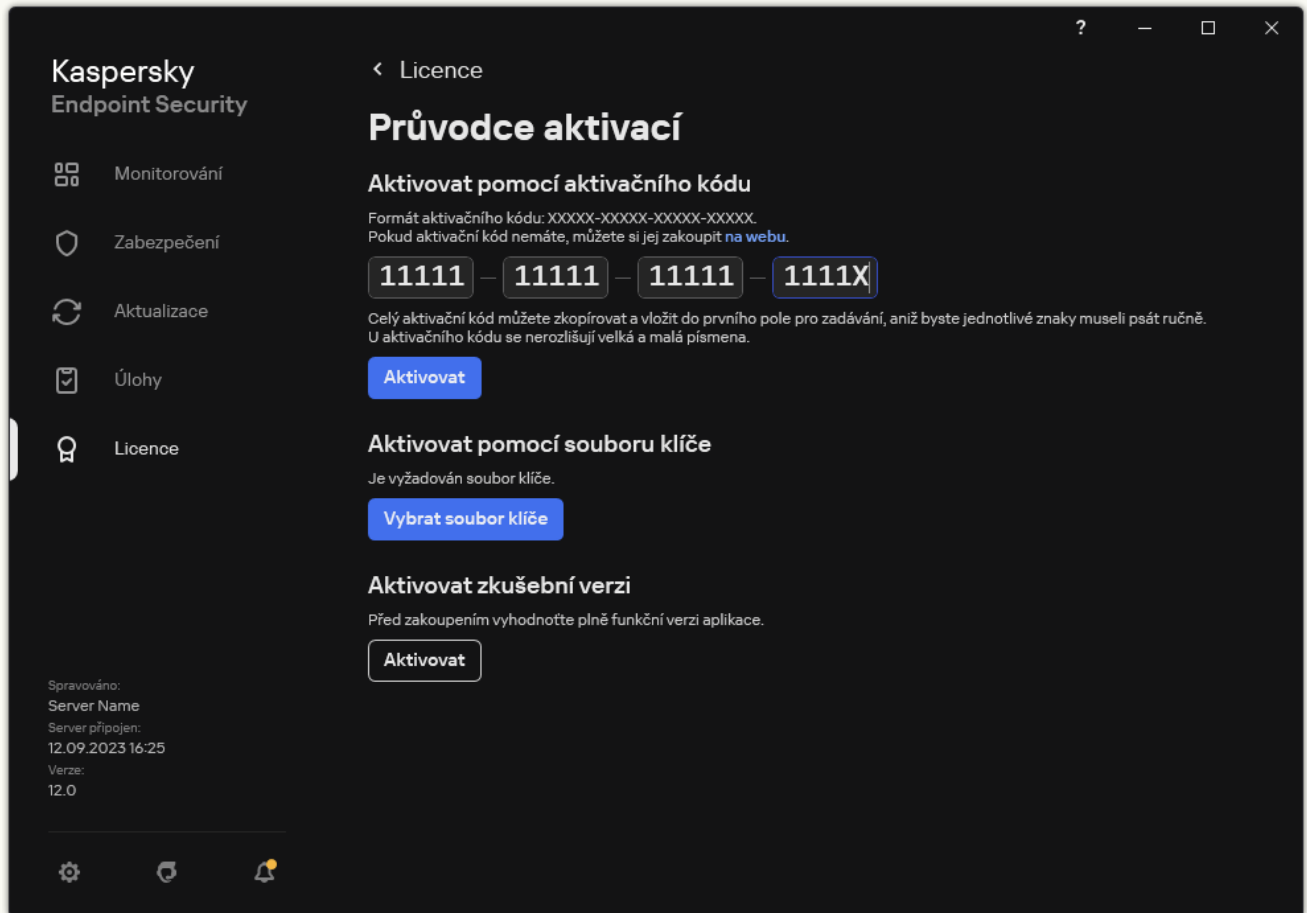
Aktivace aplikace
