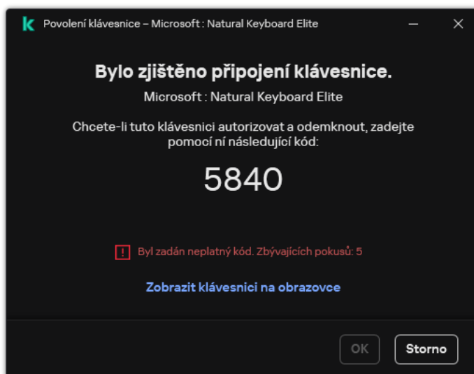
Autorizace klávesnice
