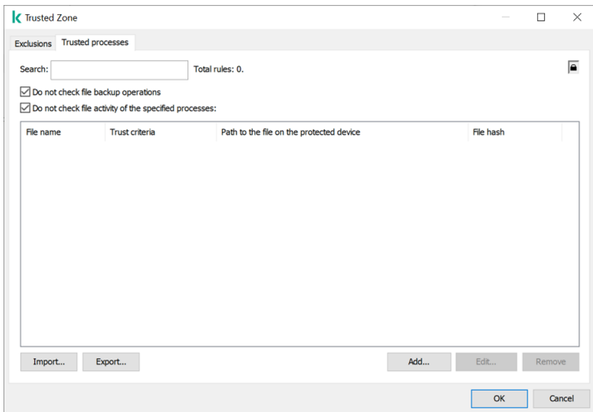
Configuración de procesos de confianza de KSWs
