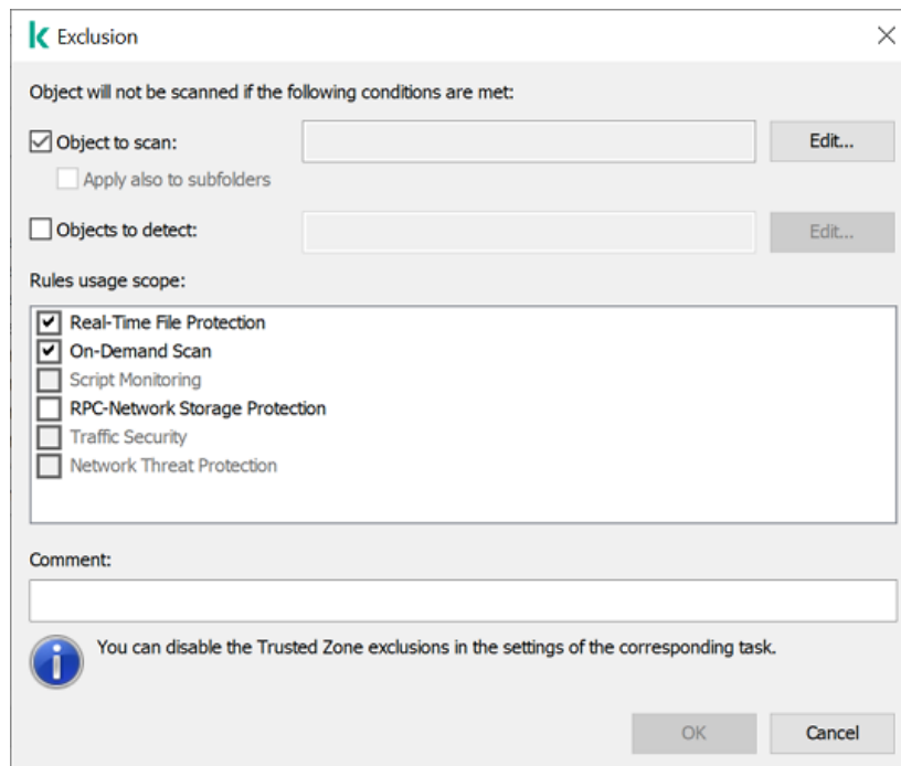
Configuración de exclusiones de KSW
