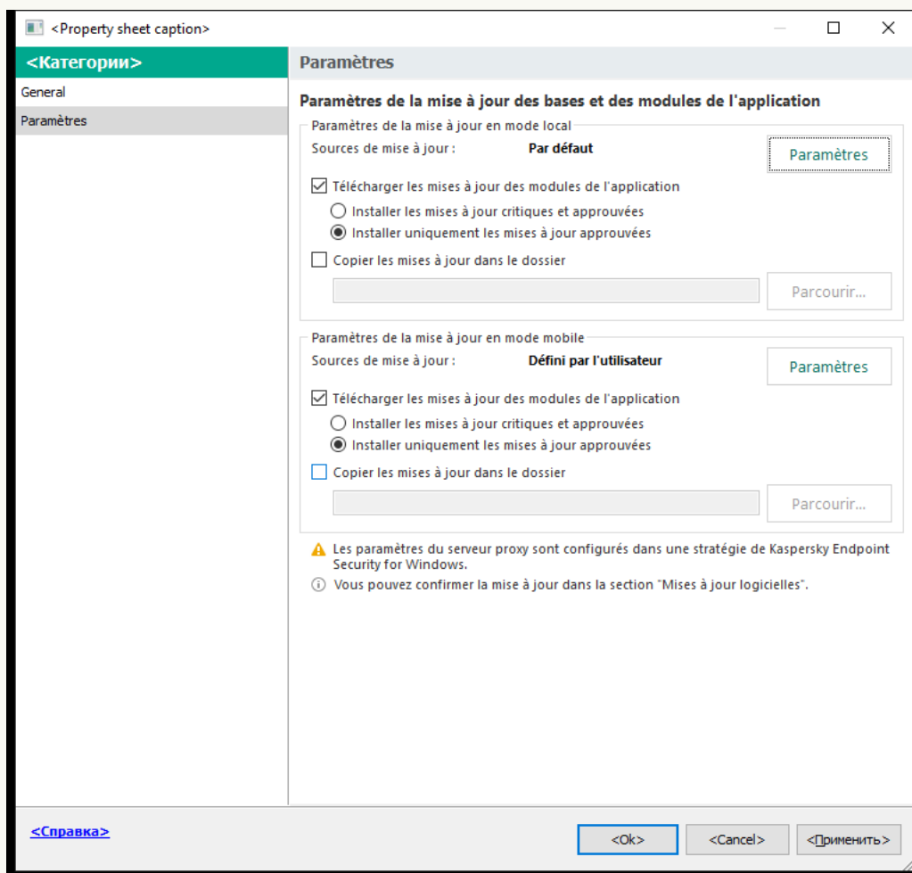
Paramètres de la tâche Mise à jour
