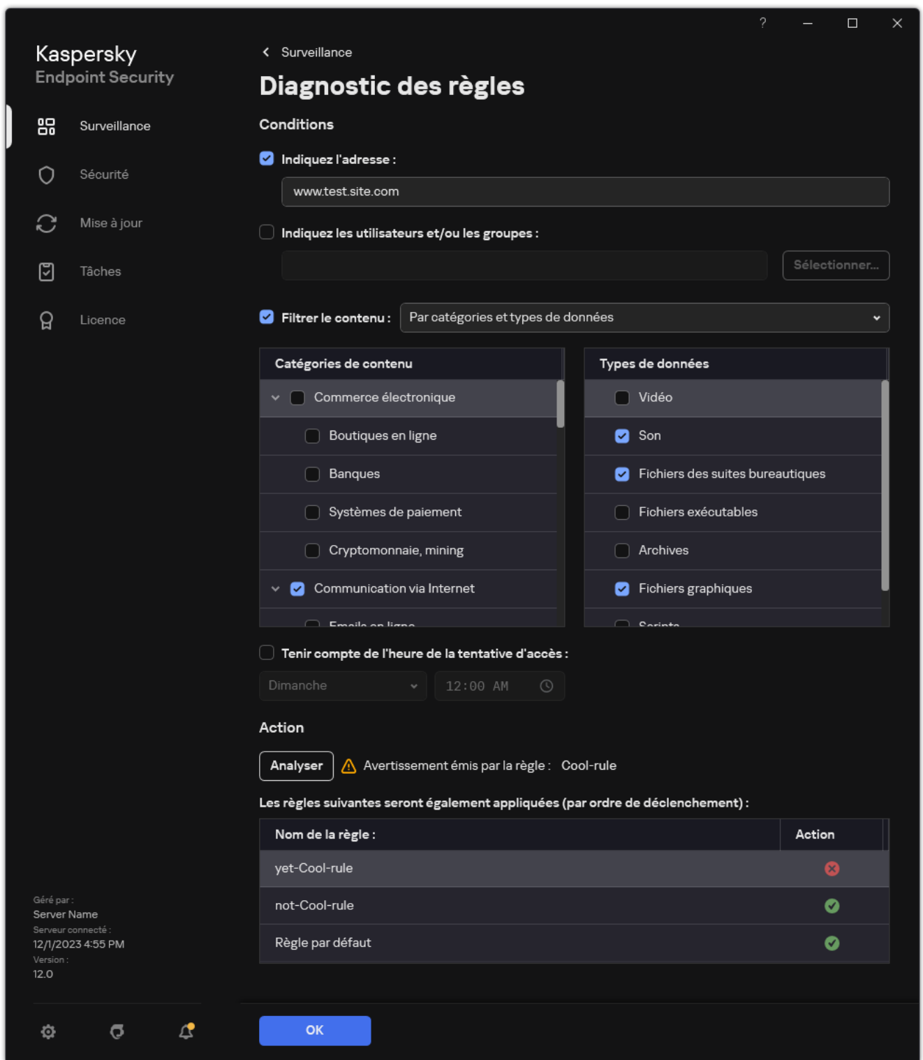
Résultat du test d'accès aux ressources Internet
