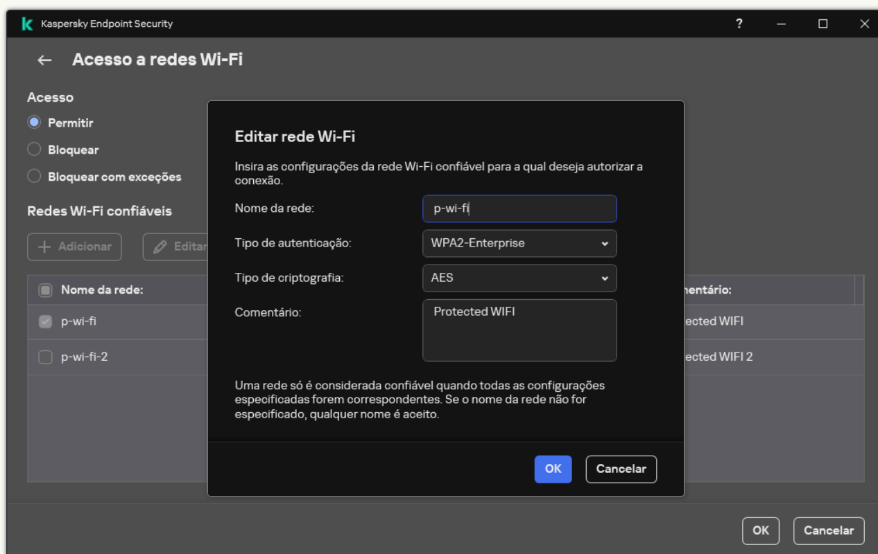
Configurações da rede Wi-Fi confiável
