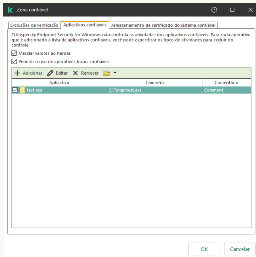
Lista de aplicativos confiáveis
