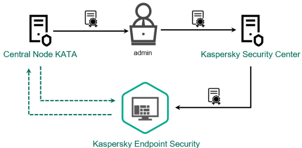
Ajouter un certificat TLS à Kaspersky Endpoint Security
