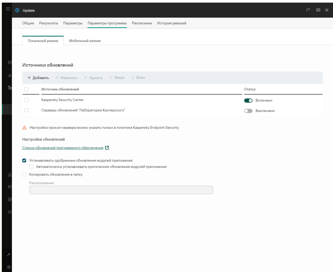
Источники обновлений
