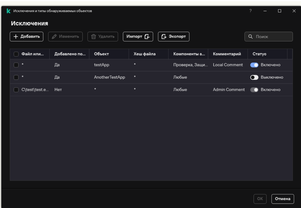
Список исключений
