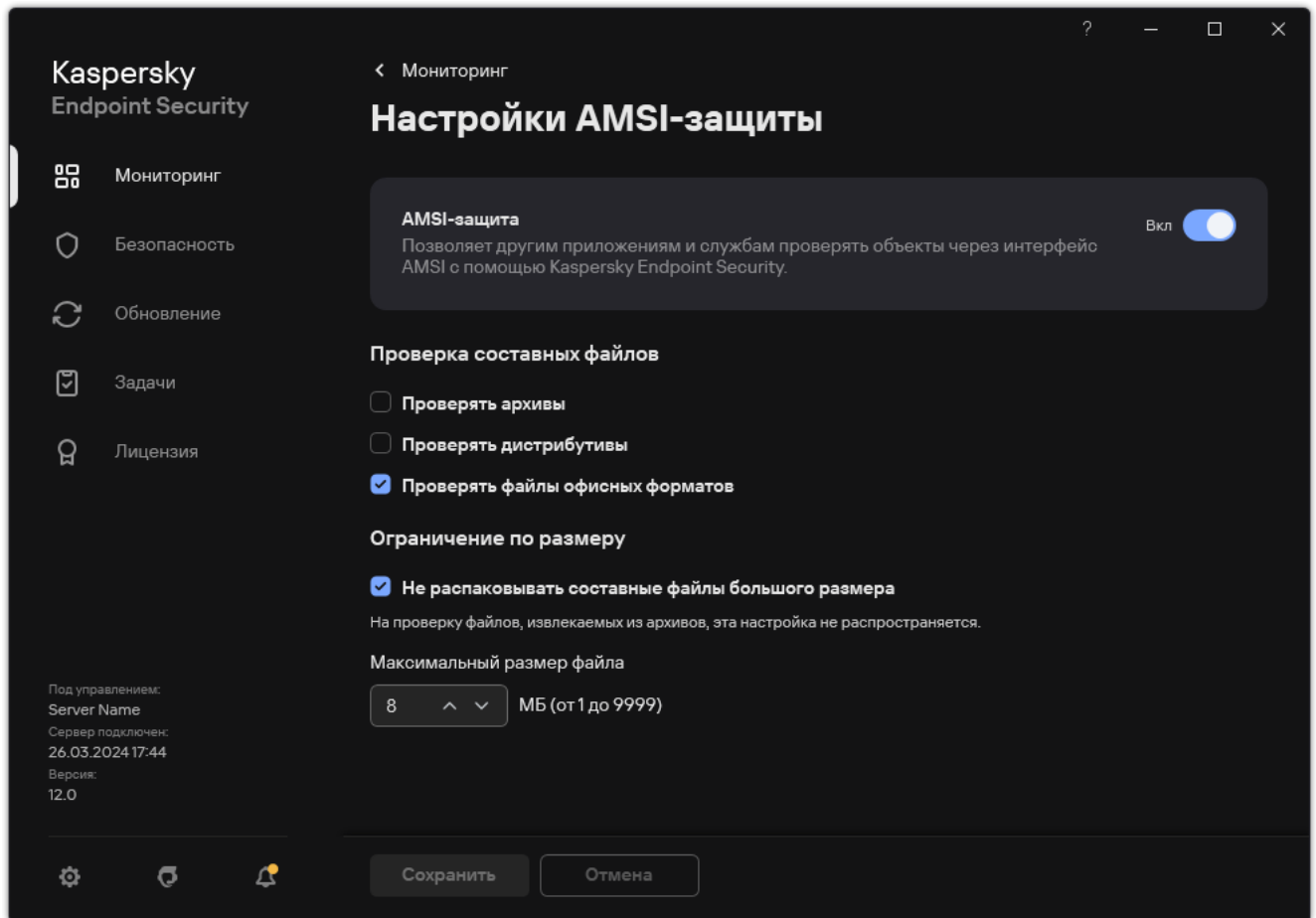
Параметры AMSI-защиты
