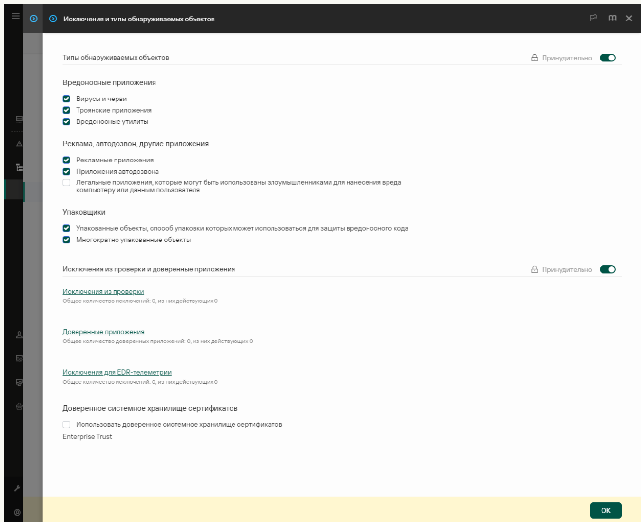
Параметры исключений
