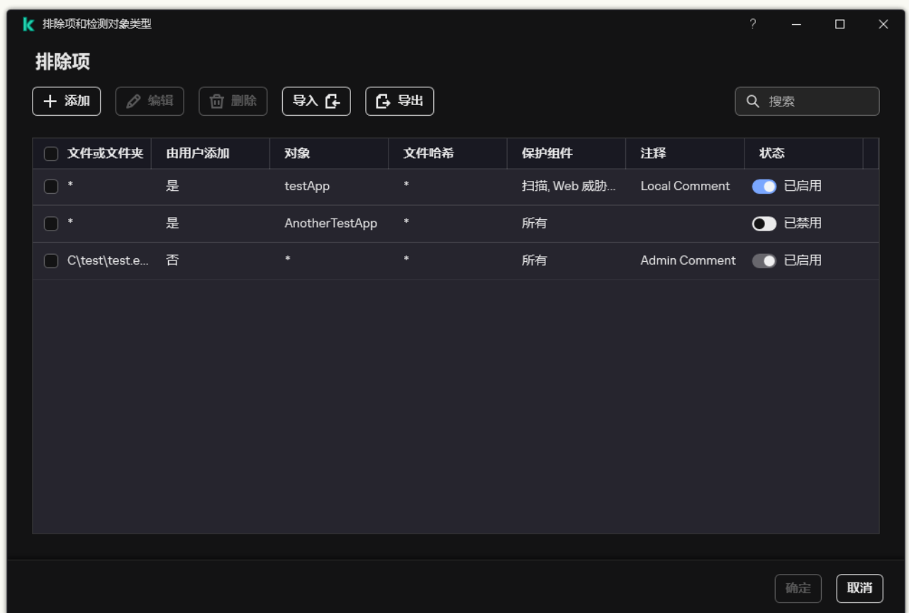
排除项列表
