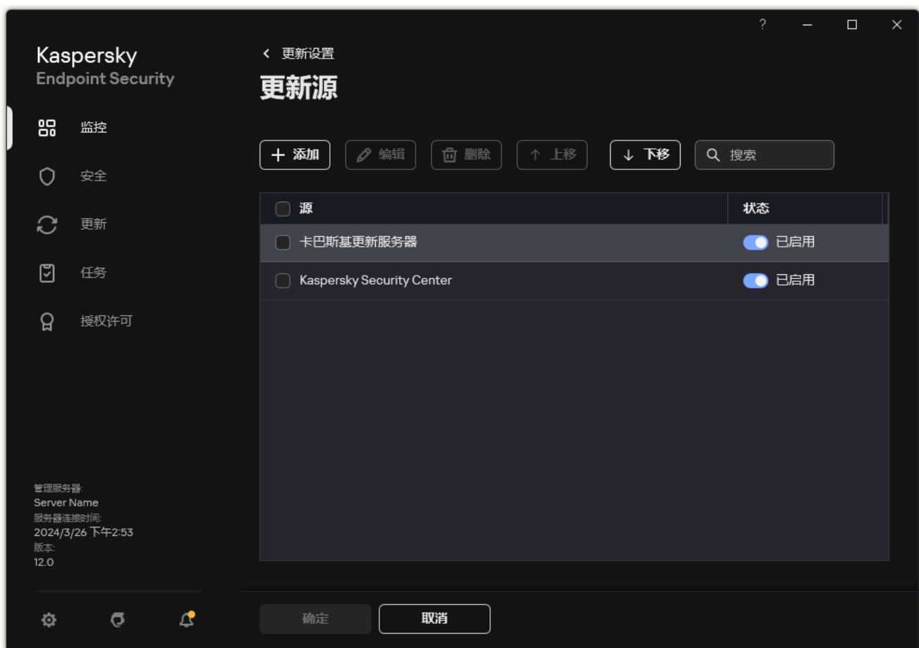
更新来源
