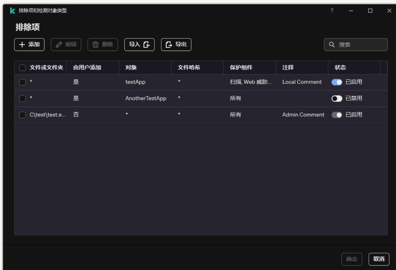
排除项列表
