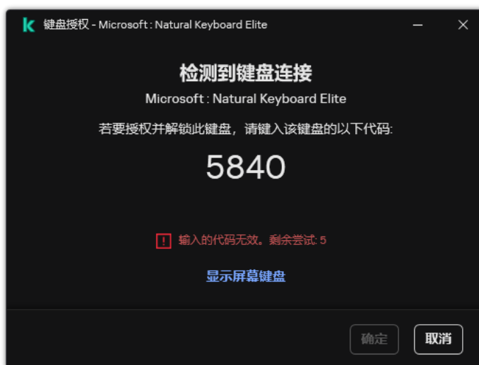
键盘授权
