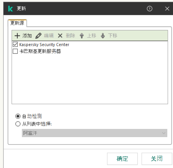
更新来源
