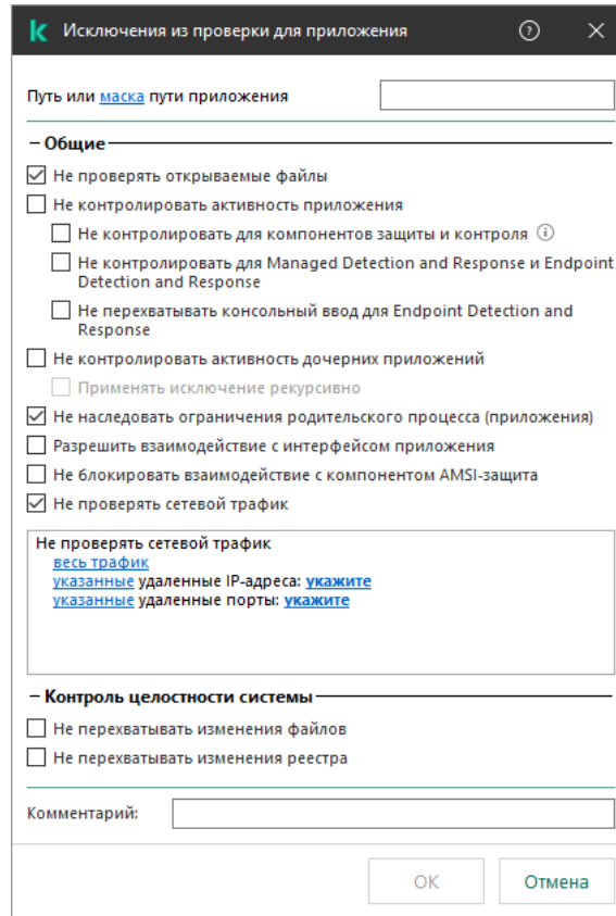
Параметры доверенного приложения KES
