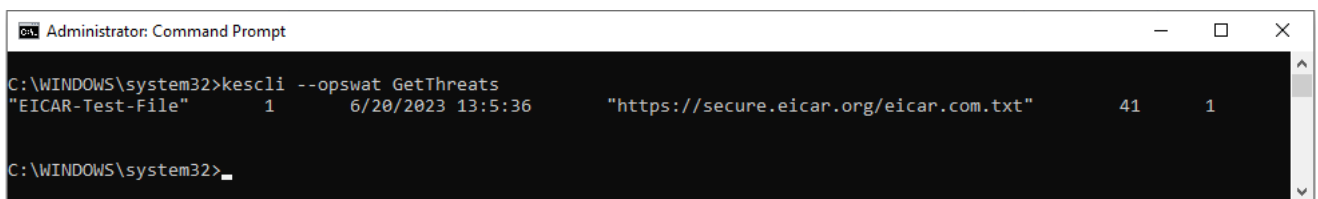
Управление приложения из командной строки
