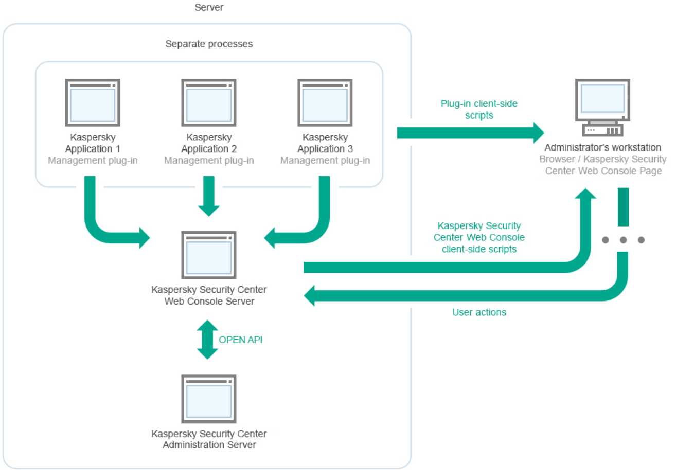
نشر مخطط خادم إدارة Kaspersky Security Center و Kaspersky Security Center 13 Web Console
