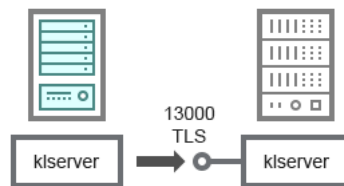
التسلسل الهرمي لخوادم الإدارة: خادم الإدارة الرئيسي وخادم الإدارة الثانوي
