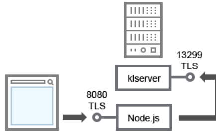
خادم الإدارة و Kaspersky Security Center 13 Web Console
