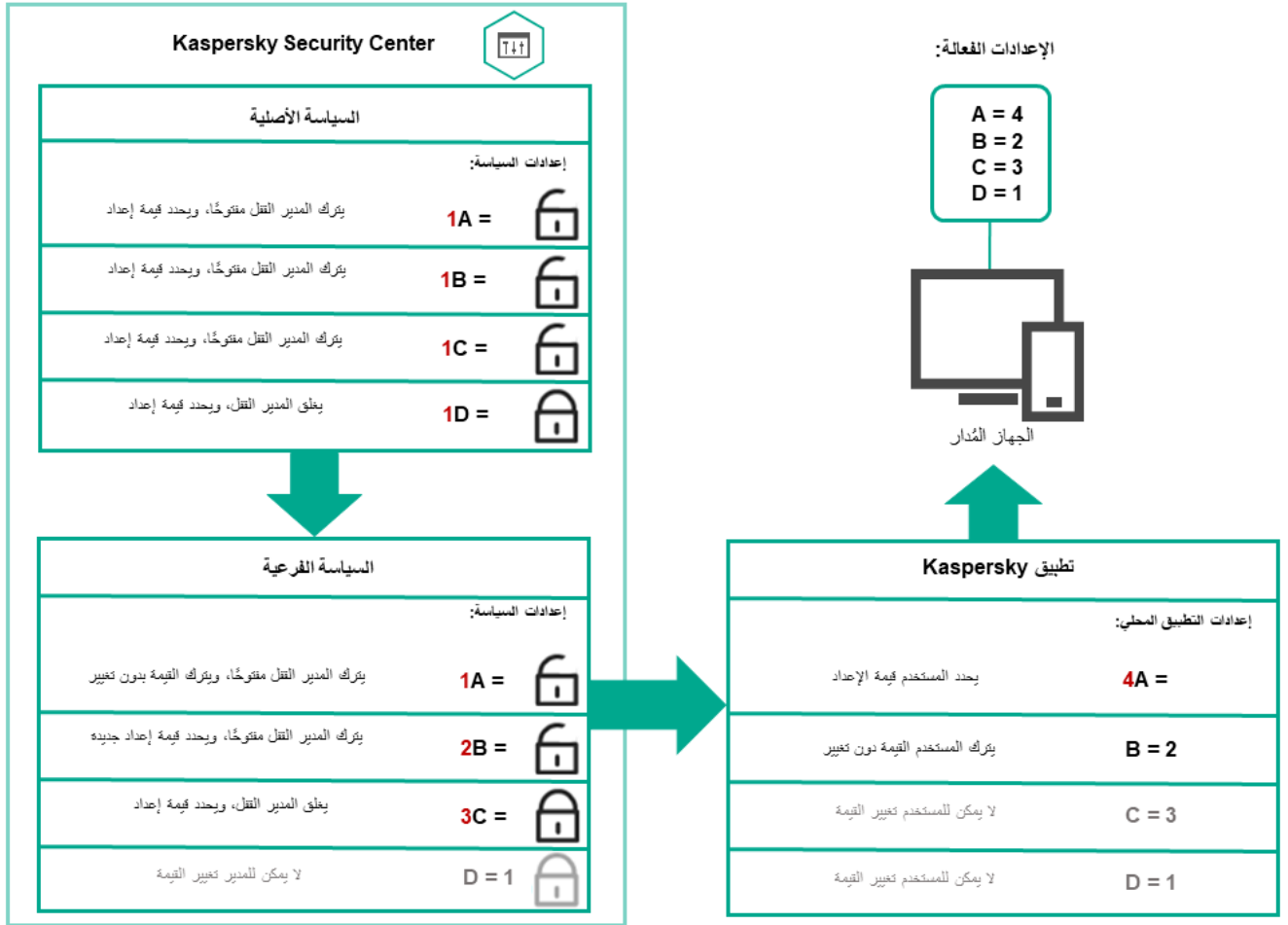
التسلسل الهرمي للسياسات
