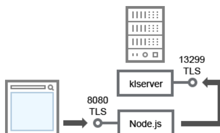
Serveur d'administration et Kaspersky Security Center 13 Web Console
