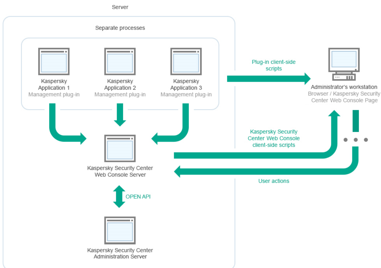
Diagramme de déploiement du Serveur d'administration de Kaspersky Security Center et de Kaspersky Security Center 13 Web Console
