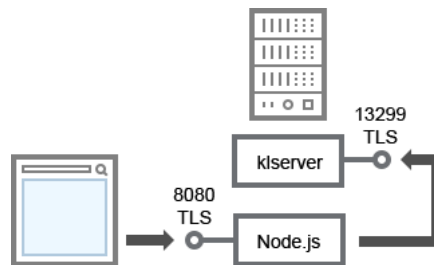
중앙 관리 서버 및 Kaspersky Security Center 13 웹 콘솔
