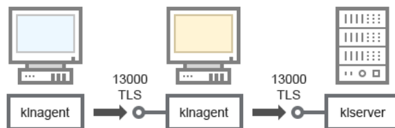
네트워크 세그먼트 및 클라이언트 기기에 연결 게이트웨이가 있는 중앙 관리 서버
