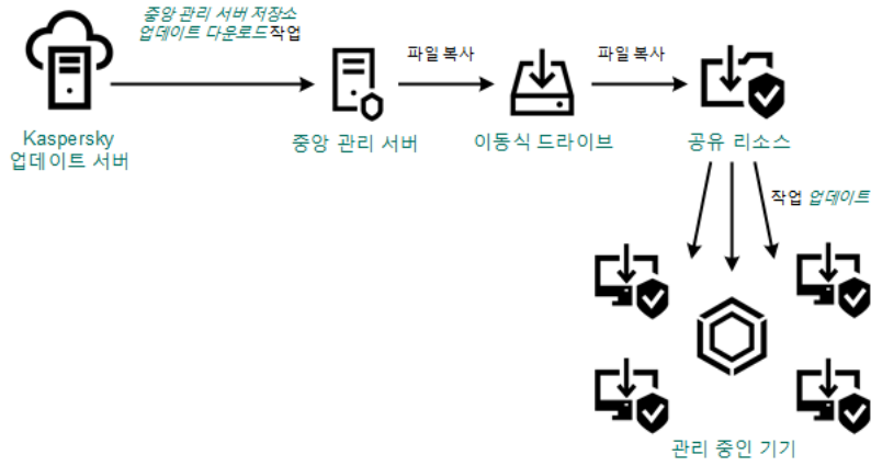
로컬 폴더, 공유 폴더 또는 FTP 서버를 통해 업데이트
