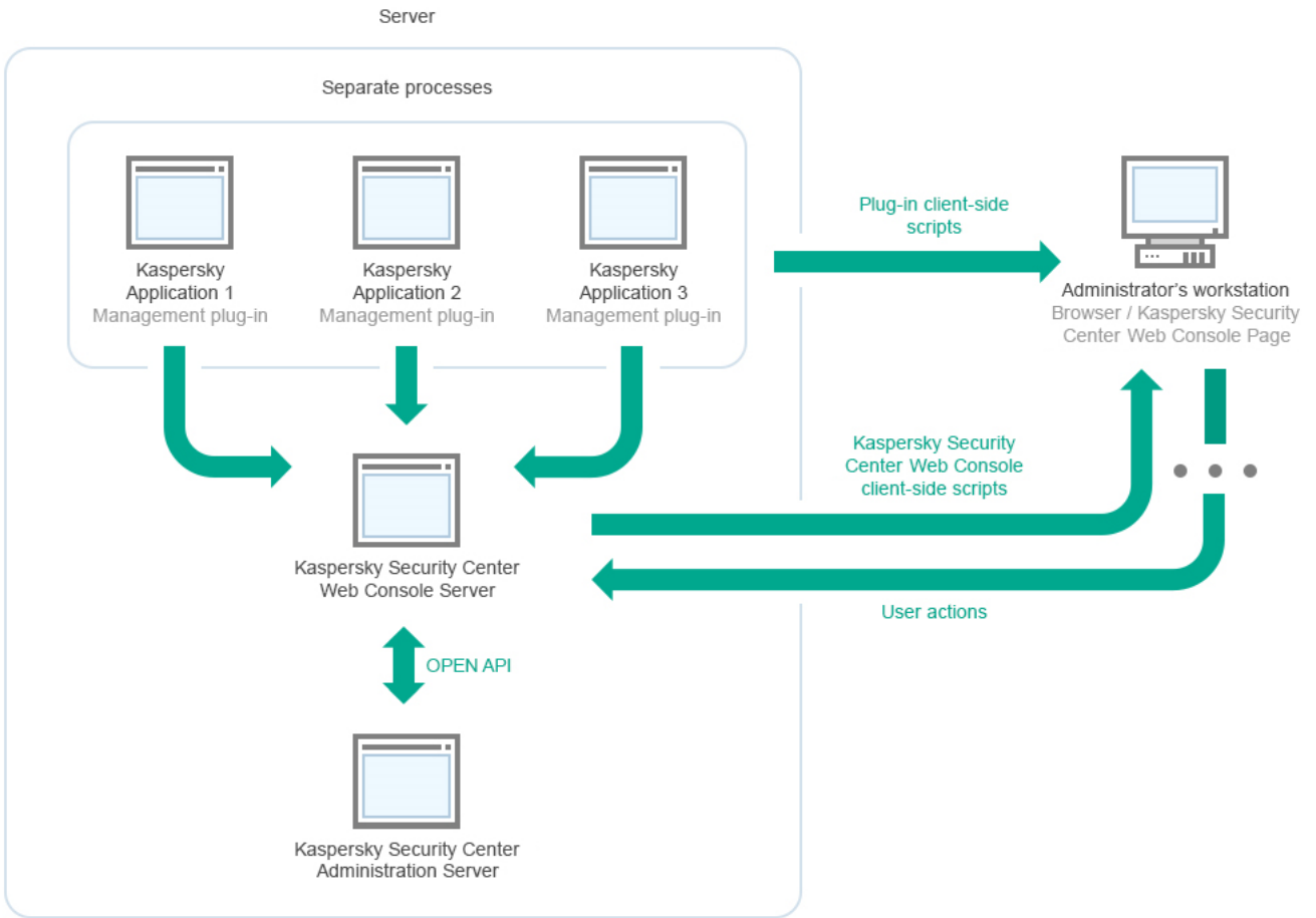
Kaspersky Security Center 중앙 관리 서버 및 Kaspersky Security Center 13 웹 콘솔의 배포 다이어그램
