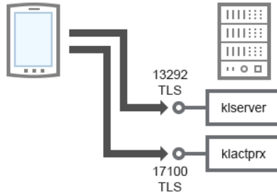
활성화 및 모바일 기기에 있는 보안 제품 관리
