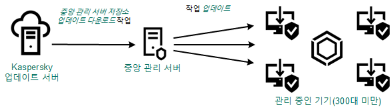
배포 지점이 없는 중앙 관리 서버 저장소 업데이트 다운로드 작업을 사용하여 업데이트
