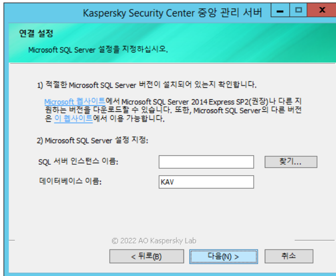
Microsoft SQL Server용 연결 설정 창의 예
