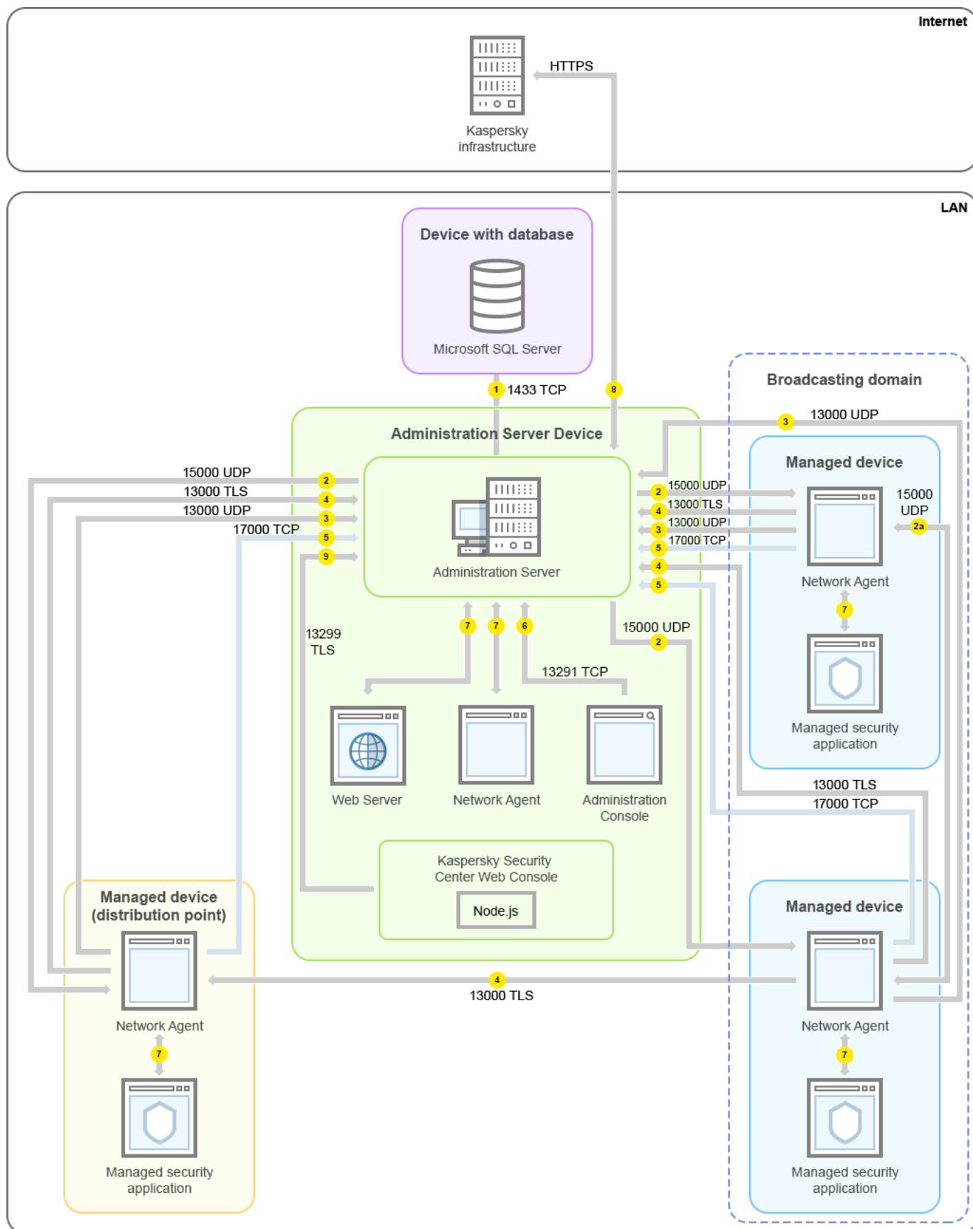
Server administracyjny i zarządzane urządzenia w sieci lokalnej (LAN)
