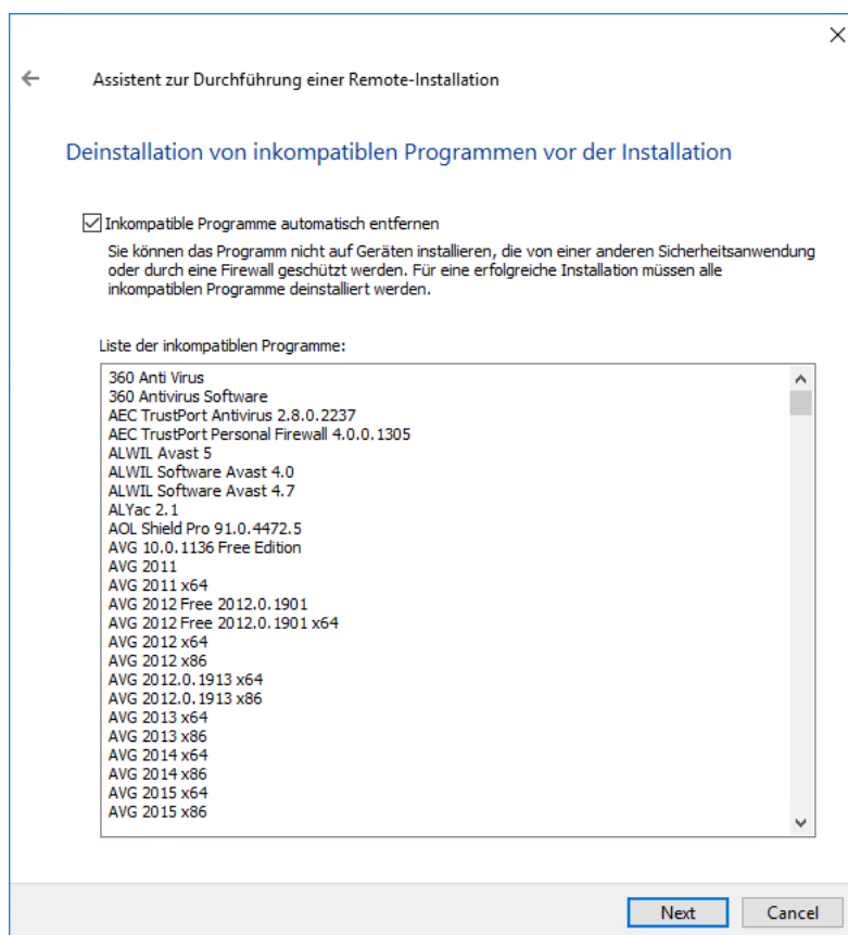
Liste mit inkompatiblen Programmen, die im Assistenten zur Durchführung einer Remote-Installation angezeigt wird.
