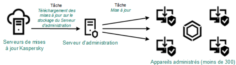
Mise à jour à l'aide de la tâche Téléchargement des mises à jour sur le stockage du Serveur d'administration sans points de distribution
