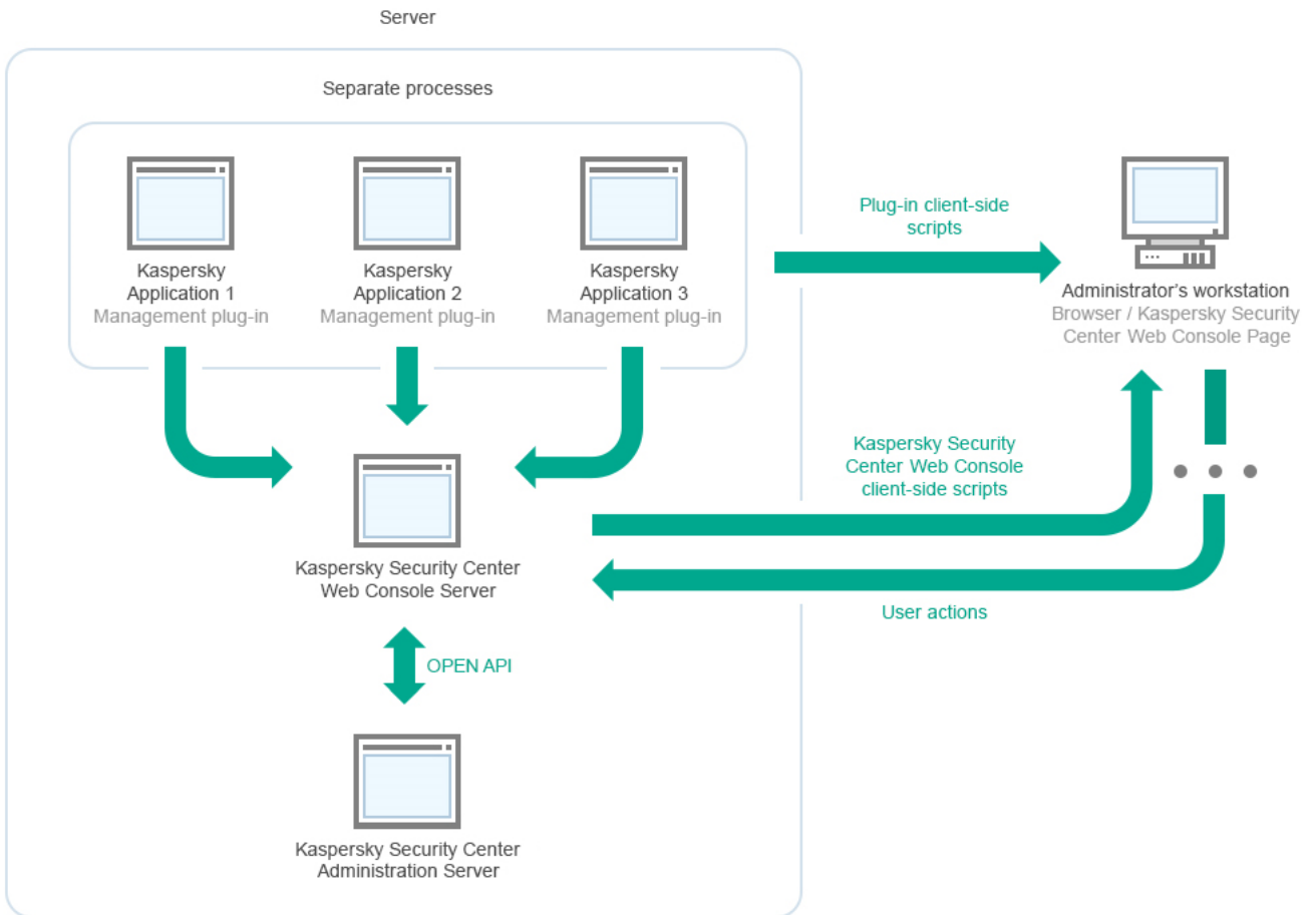
Kaspersky Security Center Linux 중앙 관리 서버 및 Kaspersky Security Center 웹 콘솔의 배포 다이어그램
