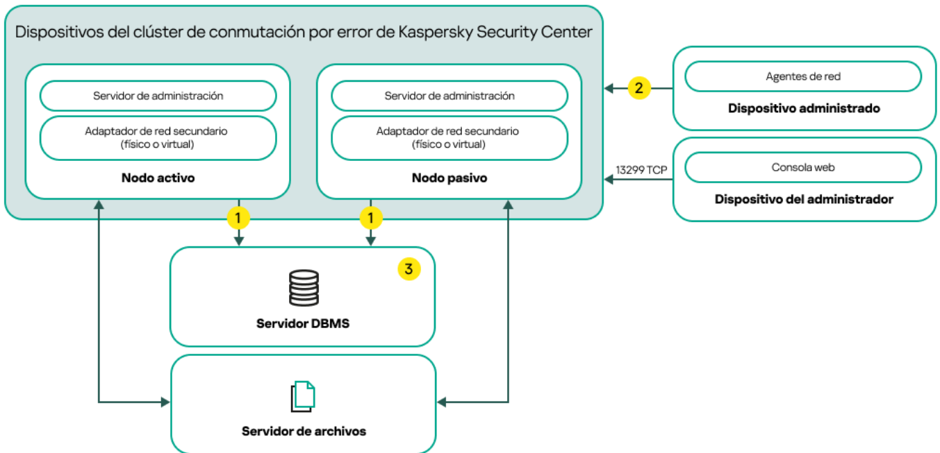
Un esquema que usa un adaptador de red secundario
