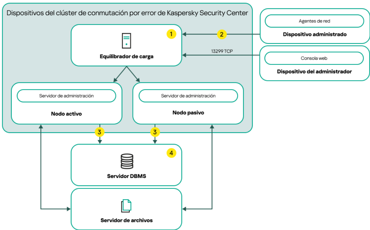
Un esquema que usa un equilibrador de carga externo
