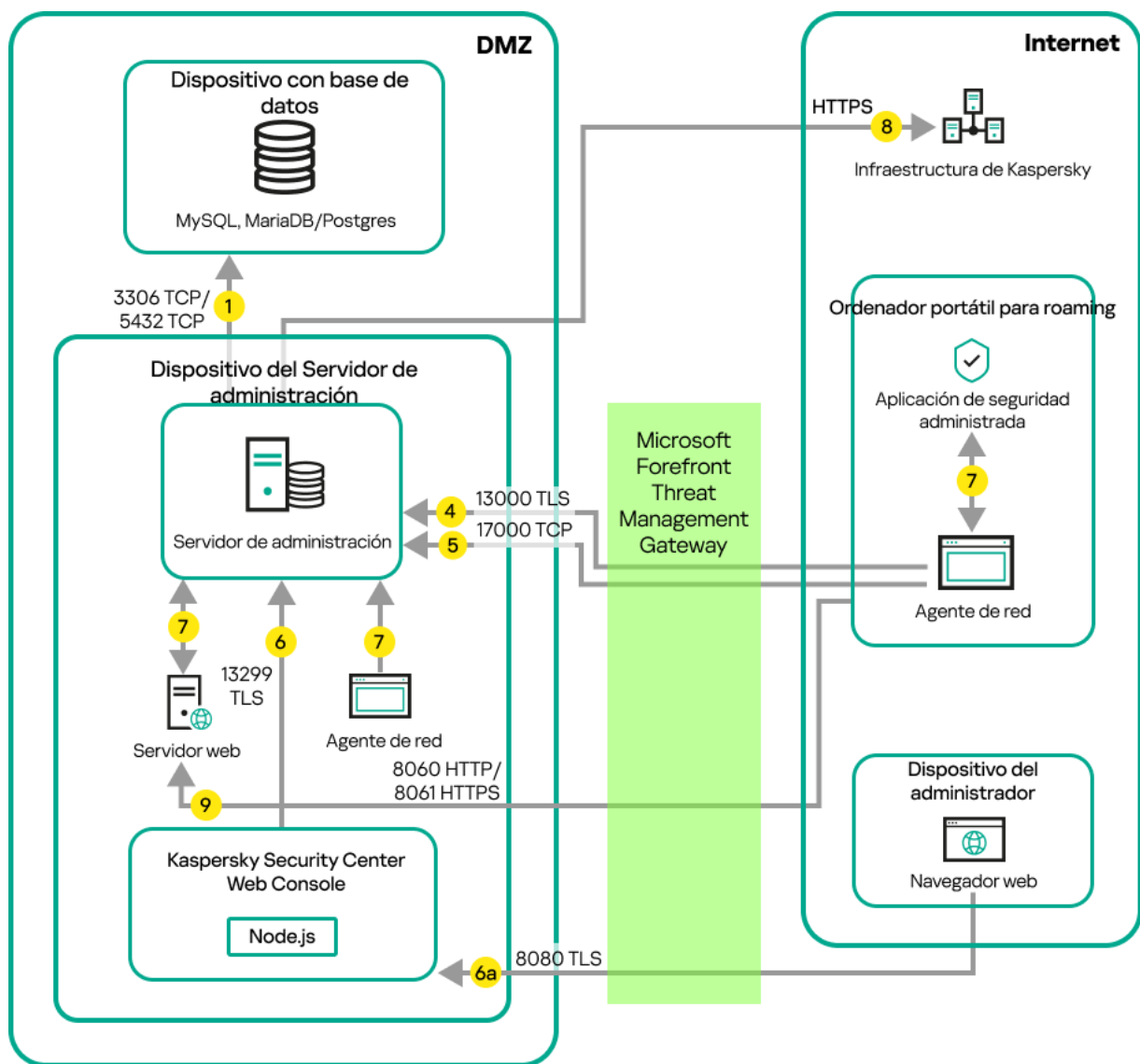
Servidor de administración en una red de área local; los dispositivos administrados se conectan al Servidor de administración a través de un firewall corporativo
