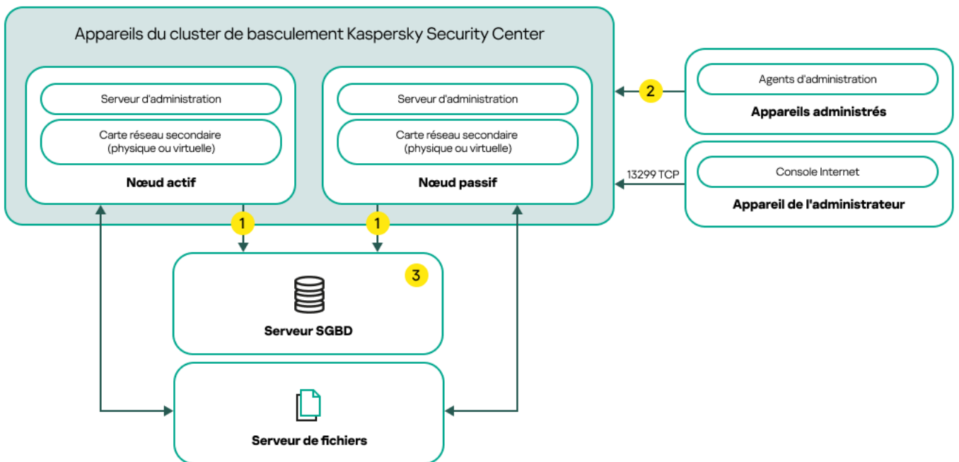
Un schéma qui utilise une carte réseau secondaire.
