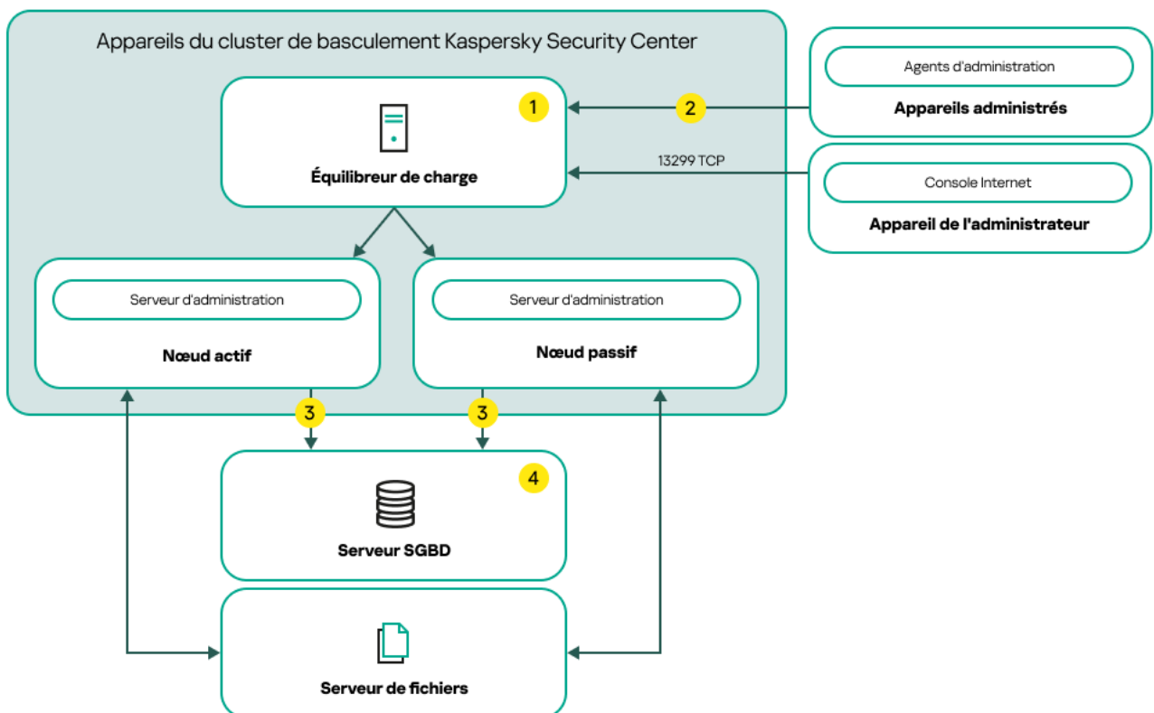
Un schéma qui utilise un équilibreur de charge tiers
