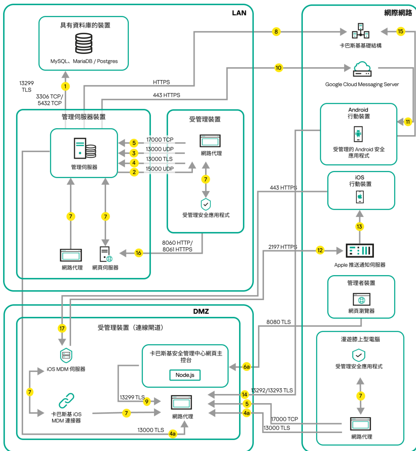
受管理行動裝置透過連線閘道器連線到管理伺服器
