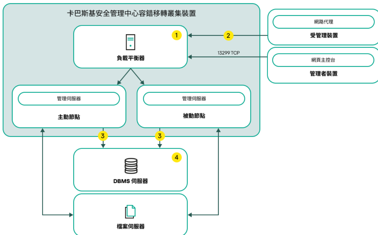
使用第三方負載平衡器和安裝在專用裝置上的 DBMS 的方案
