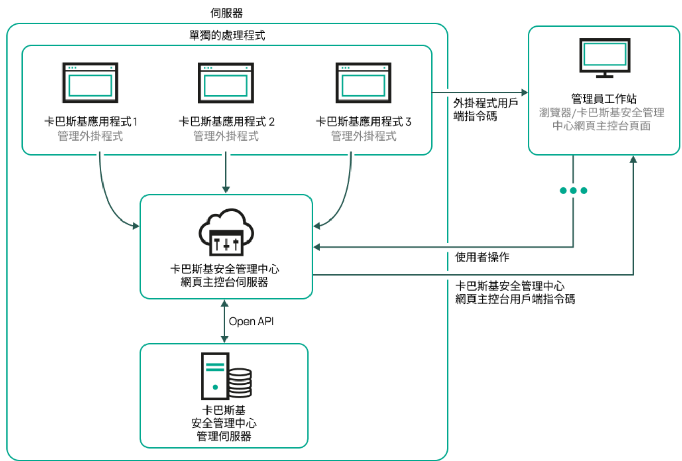
卡巴斯基安全管理中心 Linux 管理伺服器佈署圖表和卡巴斯基安全管理中心網頁主控台
