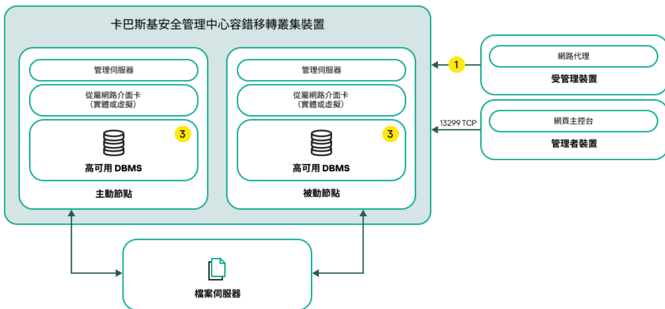
使用從屬網路介面卡和 MariaDB Galera Cluster 作為 DBMS 的方案
