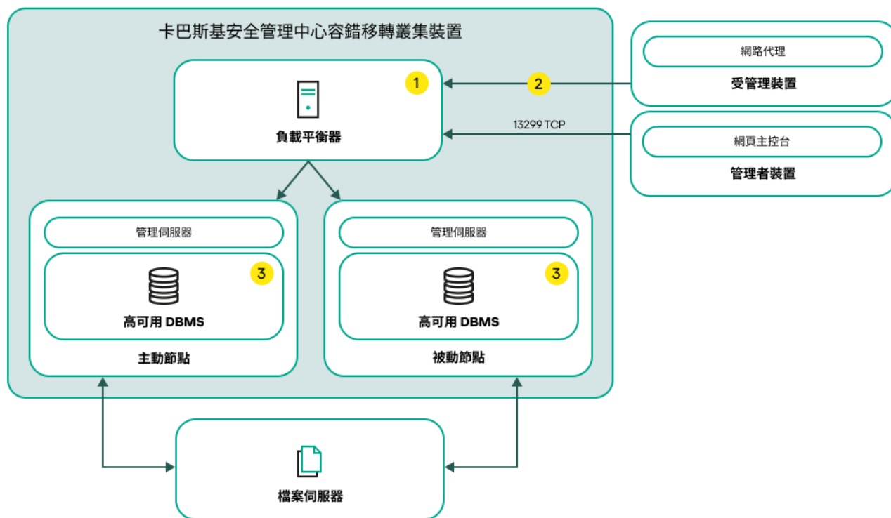
使用協力廠商負載平衡器和 MariaDB Galera Cluster 作為 DBMS 的方案
