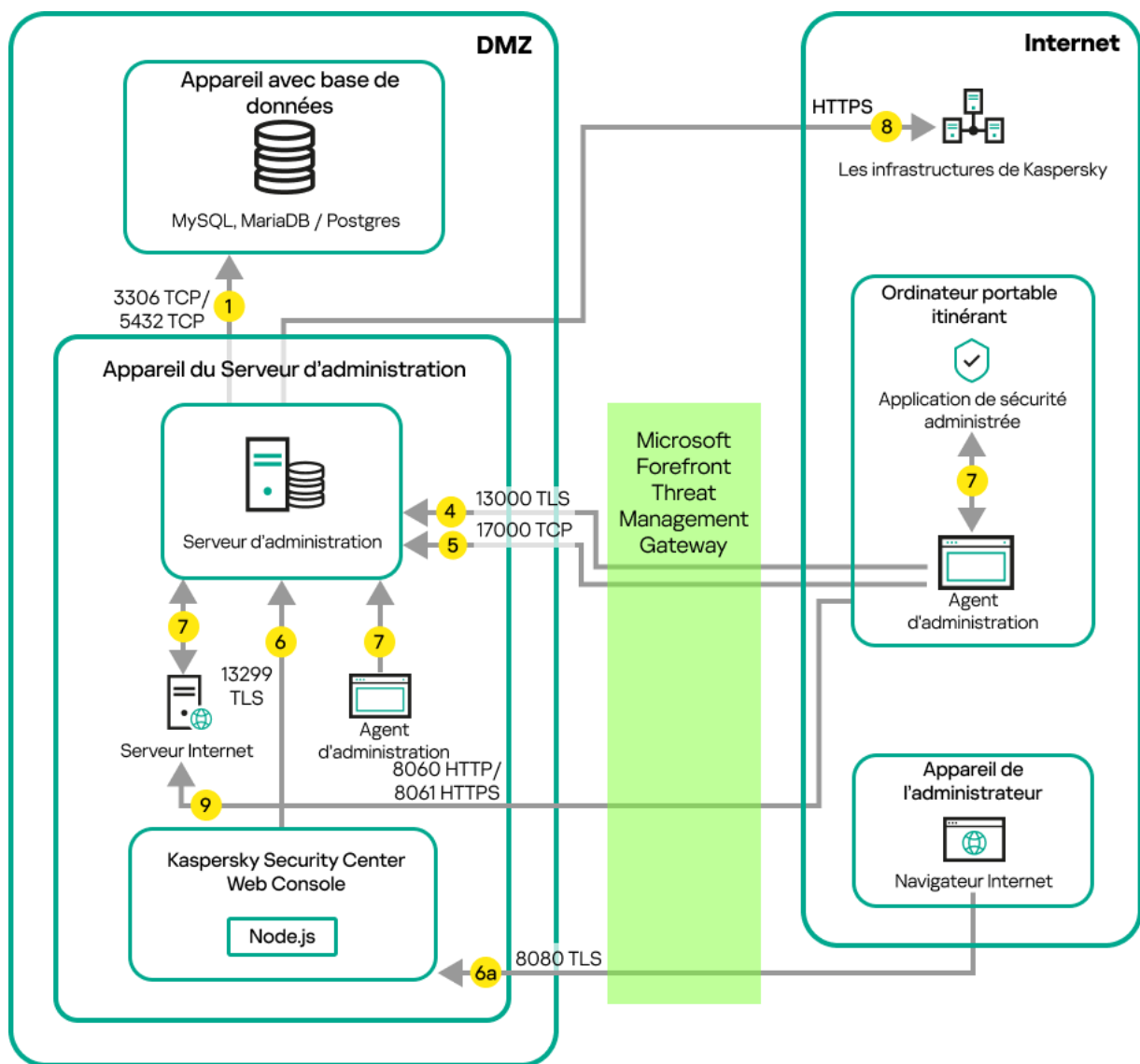
Serveur d'administration sur un réseau local ; les appareils administrés se connectent au Serveur d'administration via un pare-feu d'entreprise
