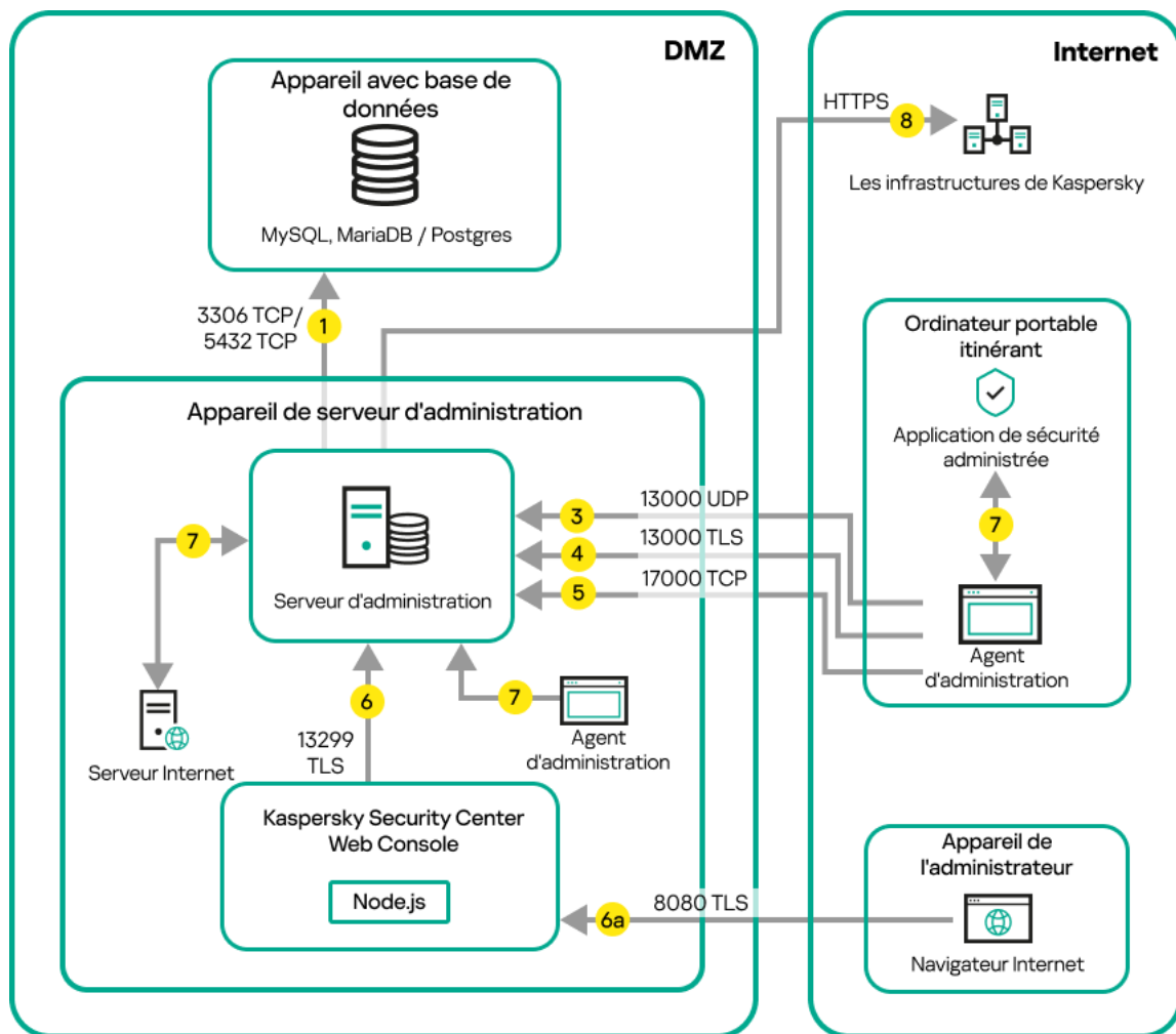
Serveur d'administration dans DMZ, appareils mobiles administrés sur Internet
