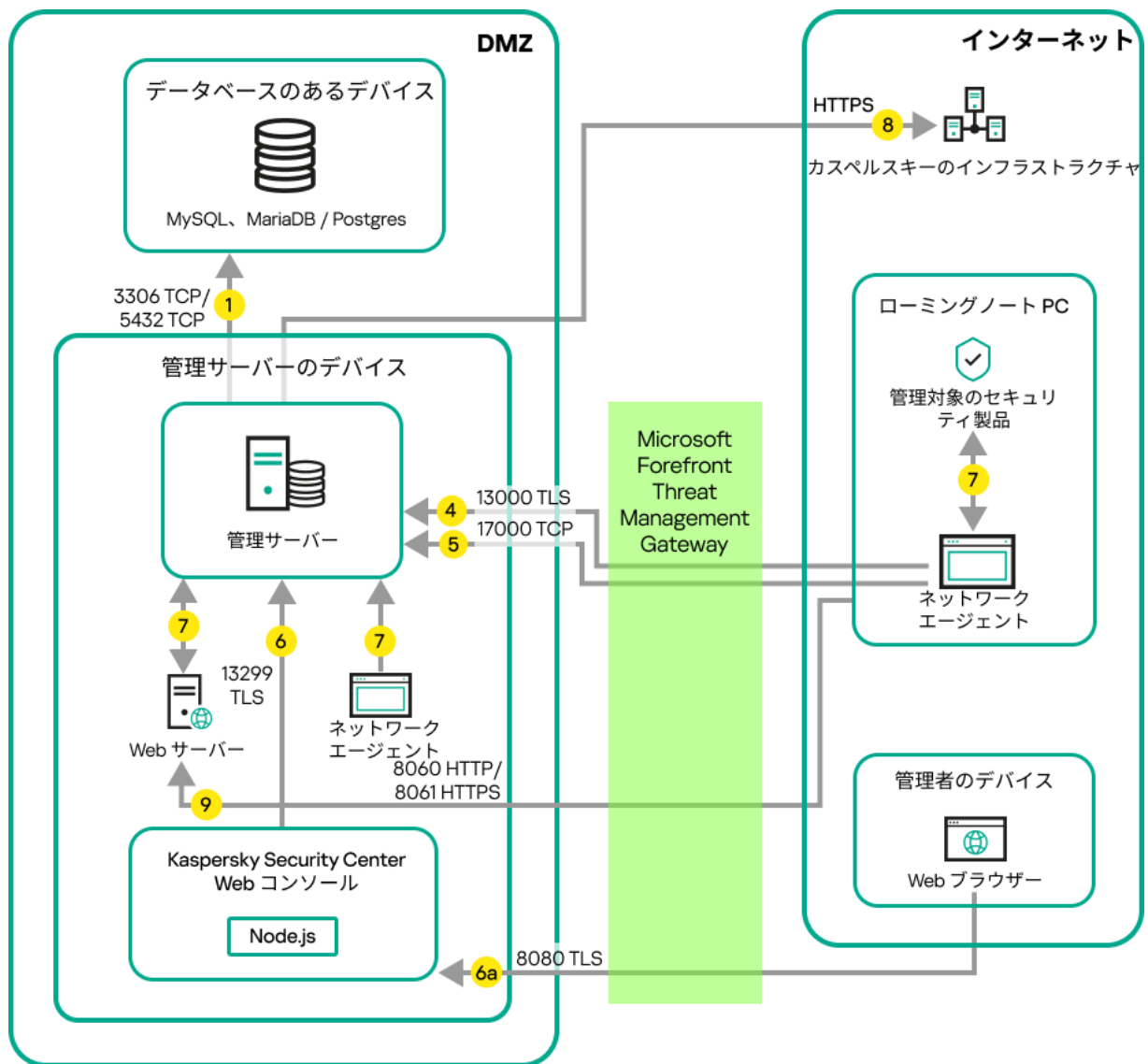
管理サーバーが LAN 内にあり、組織ネットワークのファイアウォールを経由して管理対象デバイスが管理サーバーに接続している構成
