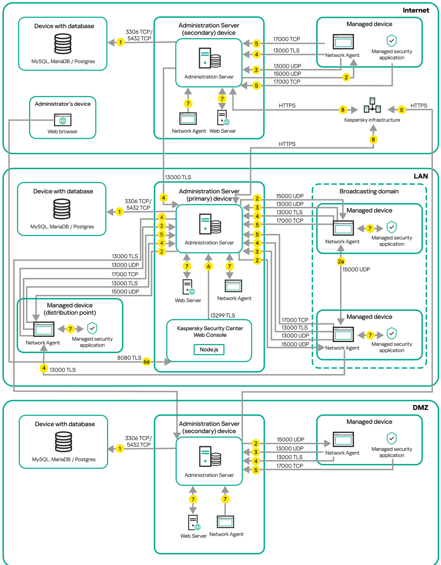
Hierarquia de Servidores de Administração: Servidor de Administração principal e dois Servidores de Administração secundários
