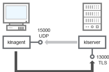
Сервер администрирования и клиентское устройство: управление программой безопасности, подключение через порт 13000 (рекомендуется)
