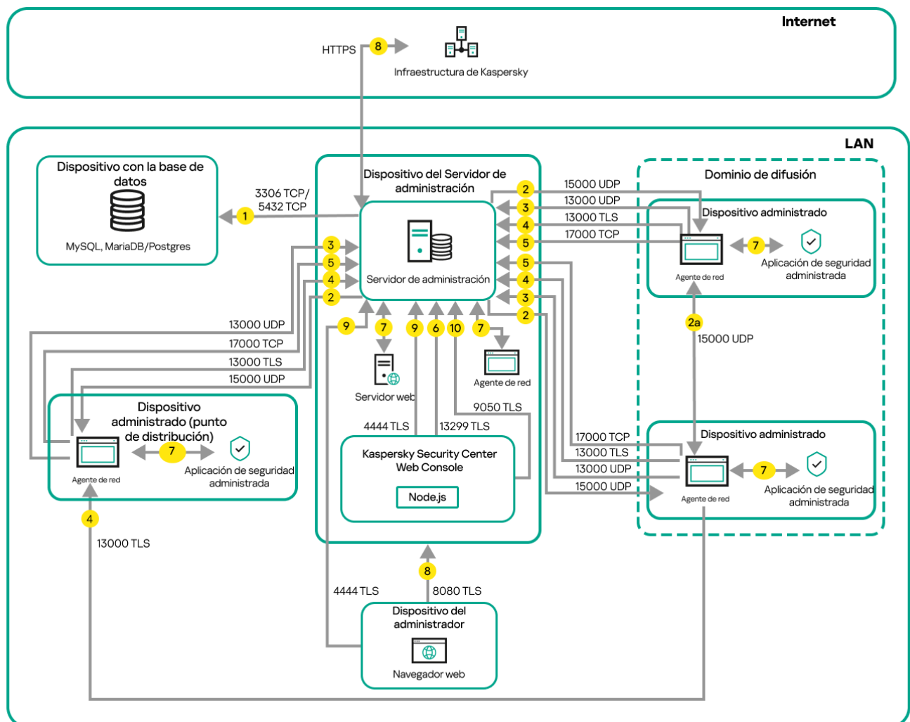
Servidor de administración y dispositivos administrados en una red de área local (LAN)
