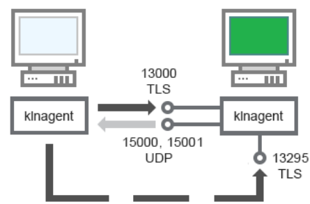
Actualización de software en un dispositivo cliente a través de un punto de distribución
