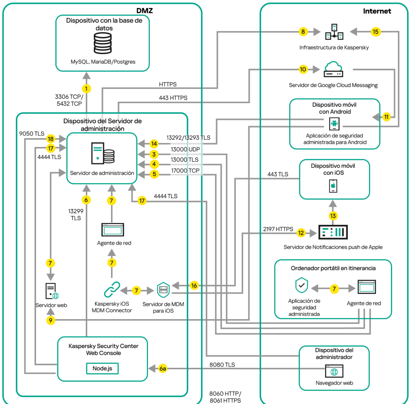
Servidor de administración en la DMZ, dispositivos móviles administrados en Internet
