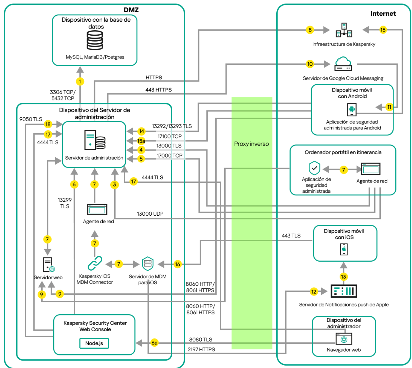
Servidor de administración en una red de área local; los dispositivos administrados se conectan al Servidor de administración a través de un proxy inverso
