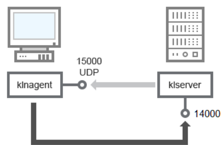
Servidor de administración y dispositivo cliente: administración de la aplicación de seguridad, conexión a través del puerto 14000 (menor seguridad)
