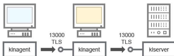
Serwer administracyjny, brama połączenia w segmencie sieci i urządzenie klienckie
