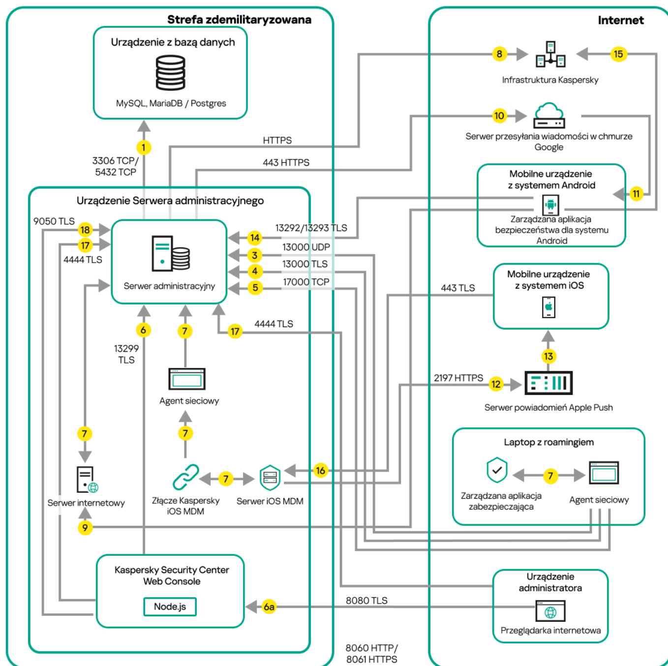
Serwer administracyjny w strefie DMZ, zarządzane urządzenia mobilne w Internecie
