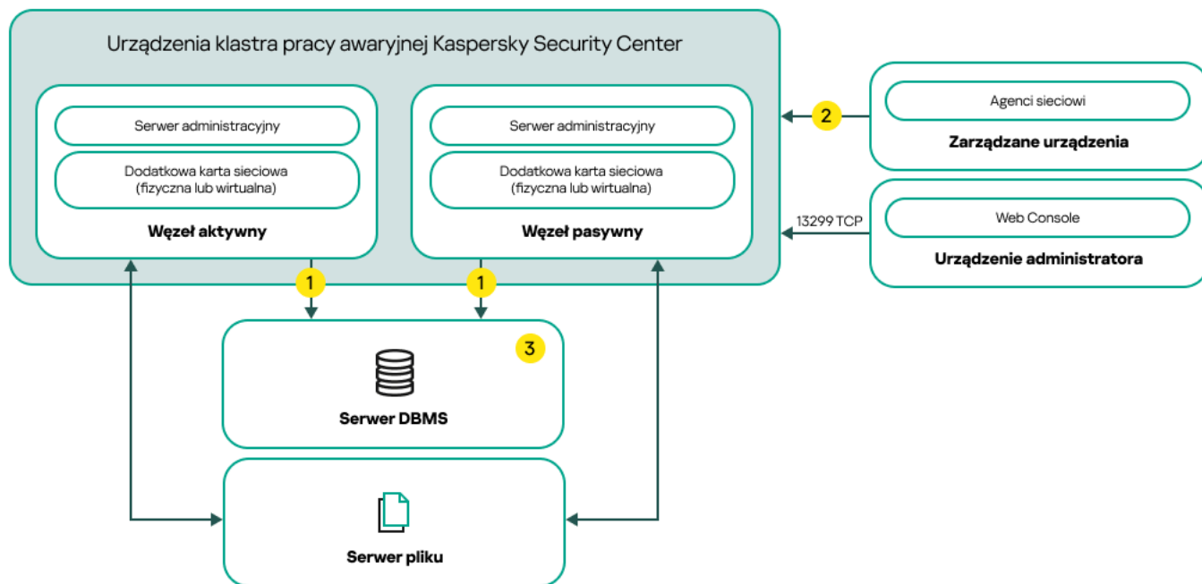
Schemat wykorzystujący dodatkową kartę sieciową i system DBMS zainstalowany na dedykowanym urządzeniu
