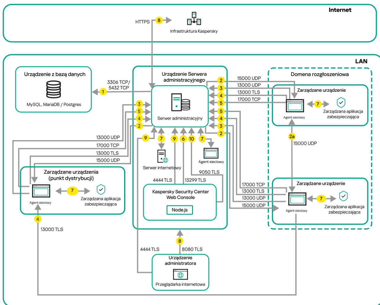
Serwer administracyjny i zarządzane urządzenia w sieci lokalnej (LAN)
