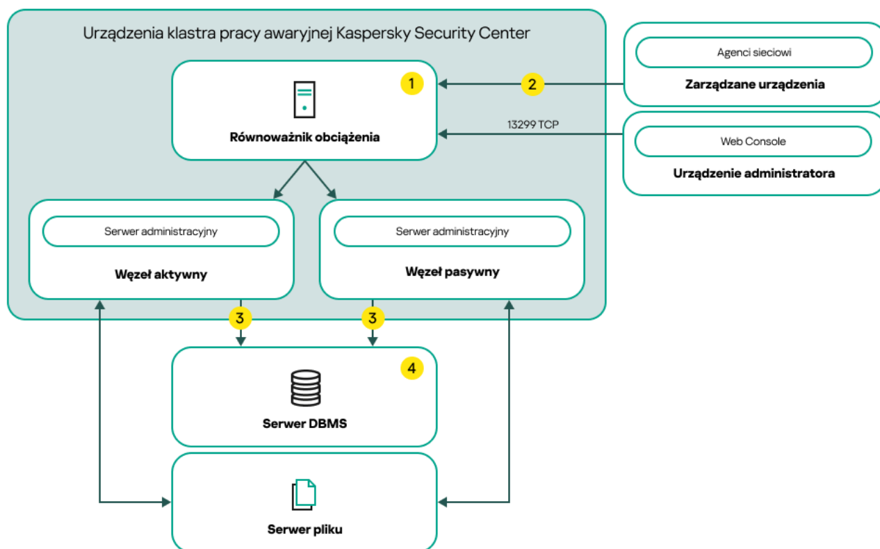
Schemat wykorzystujący zewnętrzny moduł równoważenia obciążenia i system DBMS zainstalowany na dedykowanym urządzeniu
