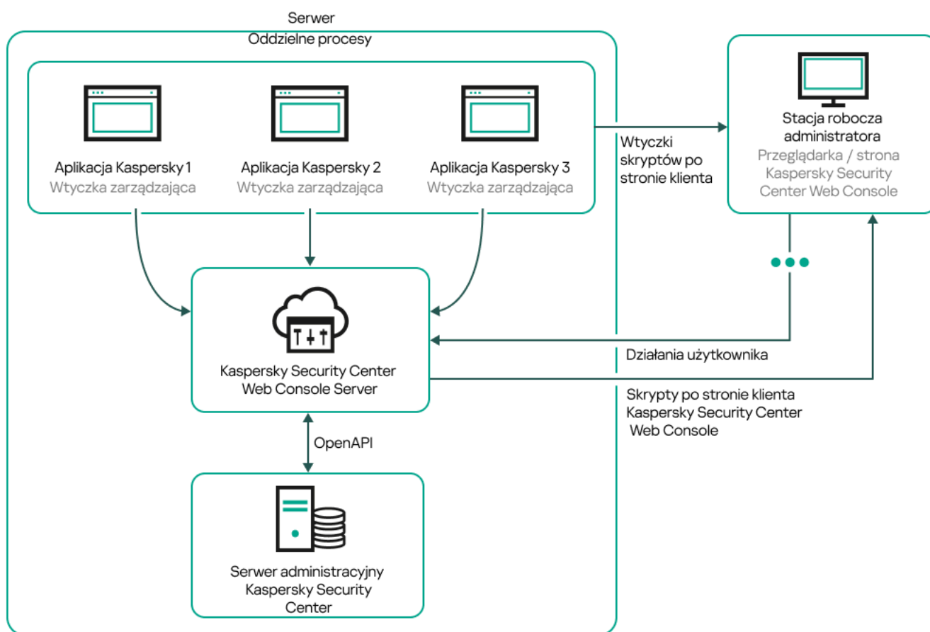
Schemat wdrożenia Serwera administracyjnego Kaspersky Security Center Linux i konsoli Kaspersky Security Center Web Console
