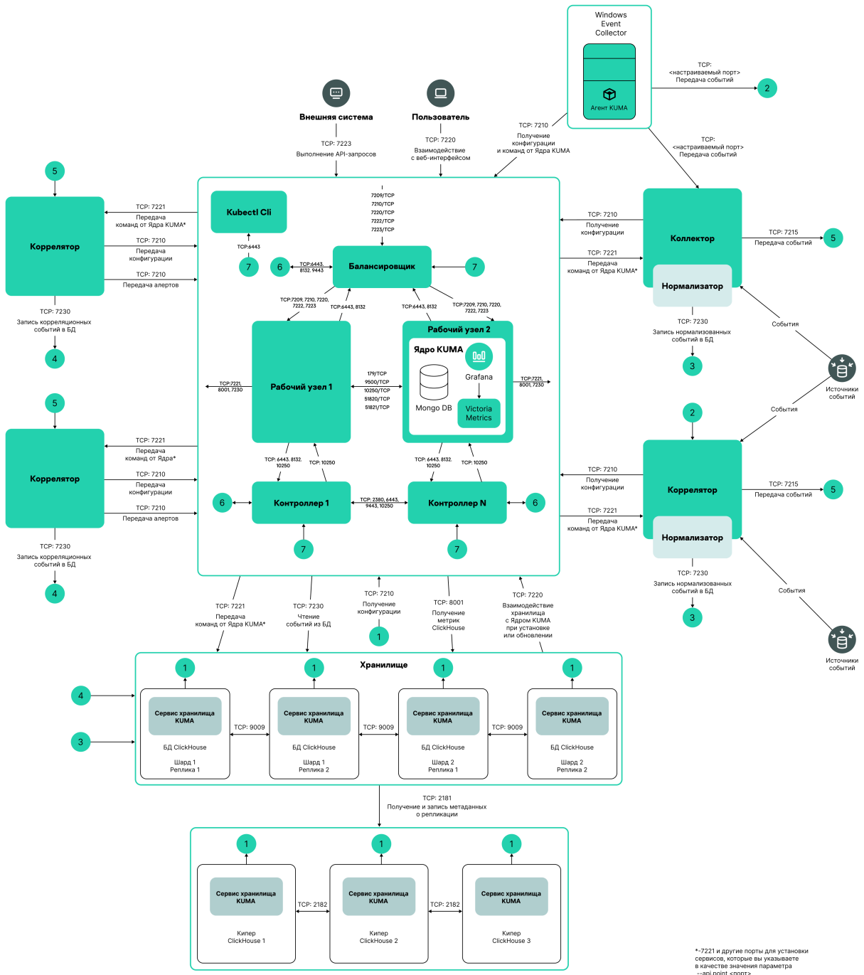
Распределенная установка в отказоустойчивой конфигурации
