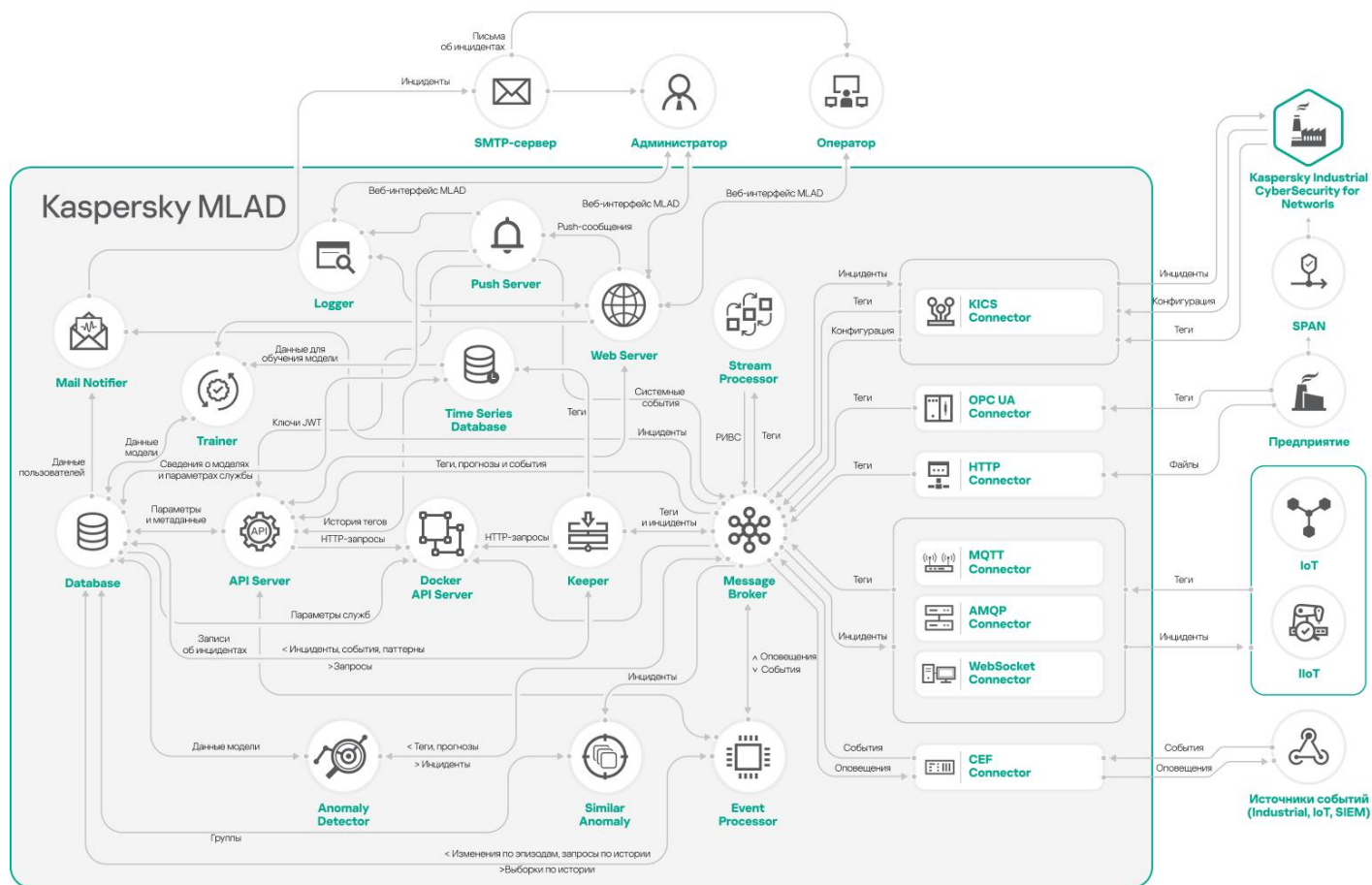
Схема взаимодействия служб Kaspersky MLAD
